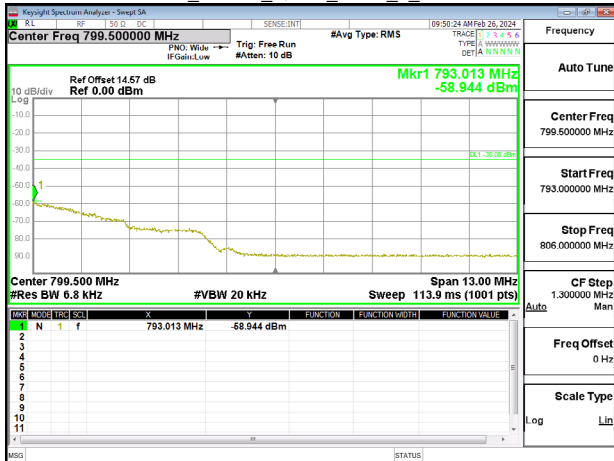
Band13_10MHz_QPSK_RB50_0_CH23230
