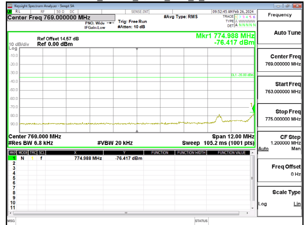
Band13_10MHz_QPSK_RB1_49_CH23230
