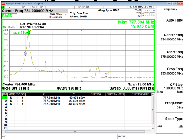
Band Edge_Band13_5MHz_QPSK_RB1_24_CH23255
