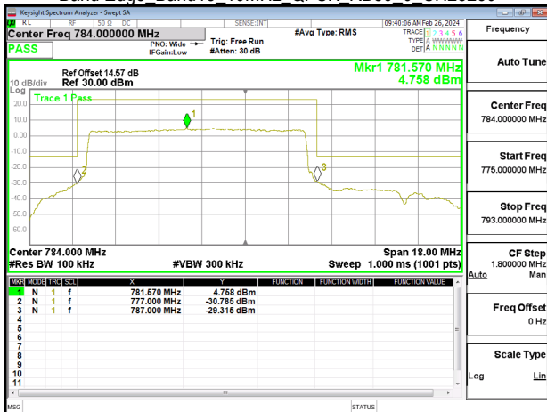
Band Edge_Band13_10MHz_QPSK_RB50_0_CH23230
