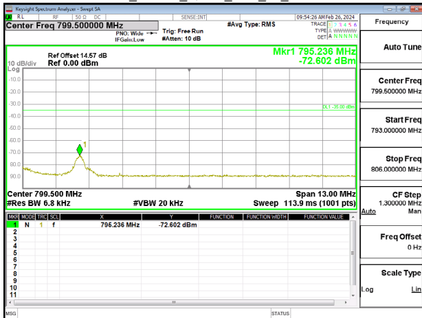
Band13_10MHz_QPSK_RB50_0_CH23230
