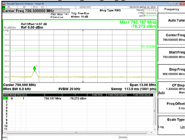
Band13_10MHz_QPSK_RB1_49_CH23230
