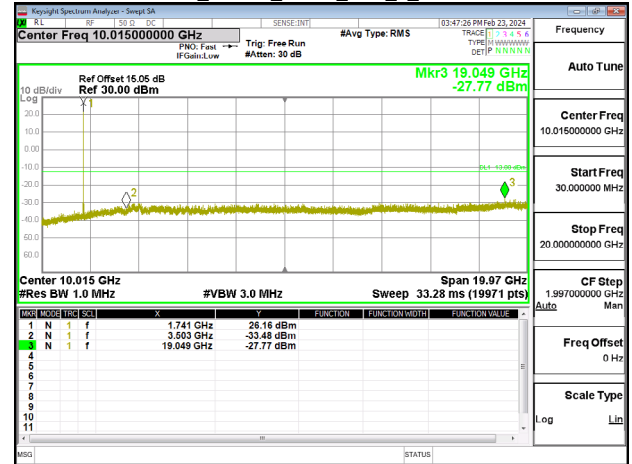
Band13_10MHz_QPSK_RB1_0_CH23230
