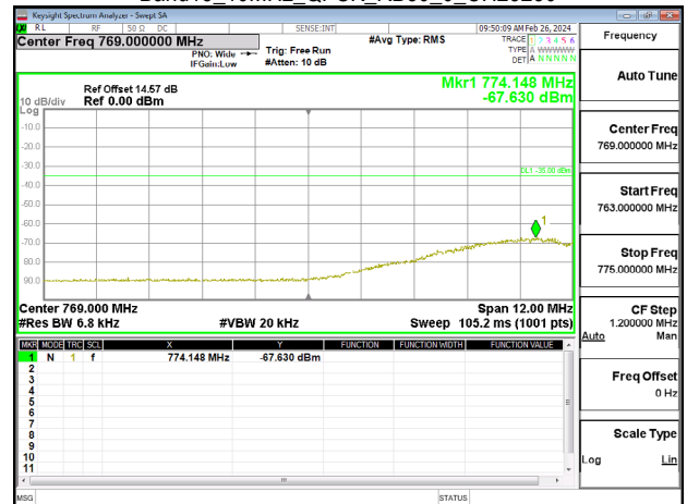
Band13_10MHz_QPSK_RB50_0_CH23230
