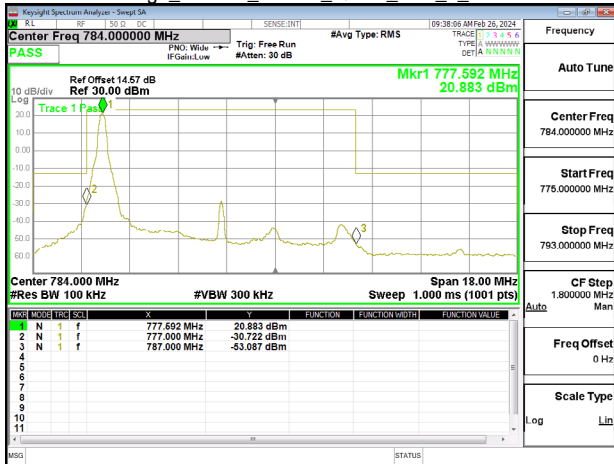
Band Edge_Band13_10MHz_QPSK_RB1_49_CH23230
