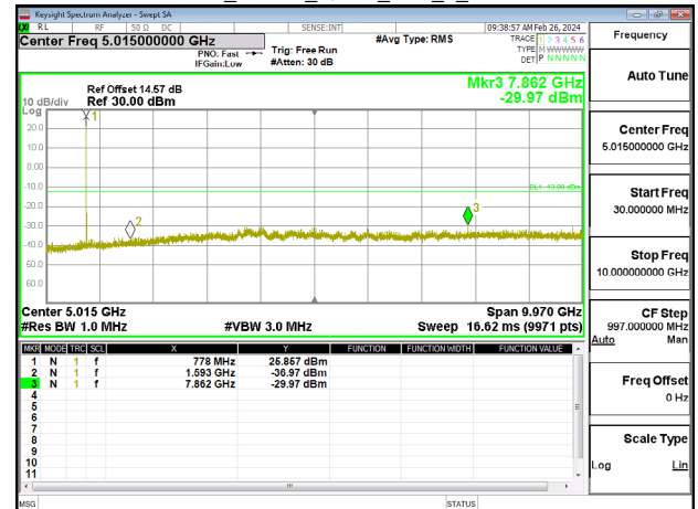
Band13_10MHz_QPSK_RB1_0_CH23230
