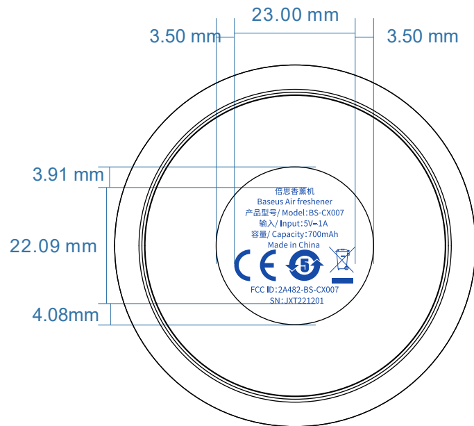
底视图
