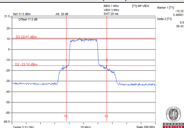
802.11ax (HE160)
