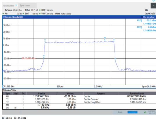
Band66-10MHz-QPSK-132022-50RB#0
