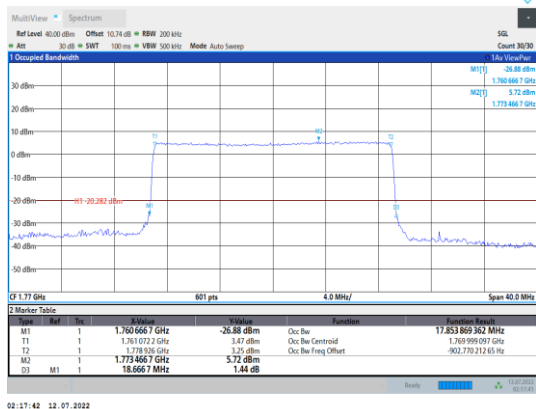
Band66-20MHz-QPSK-132572-100RB#0
