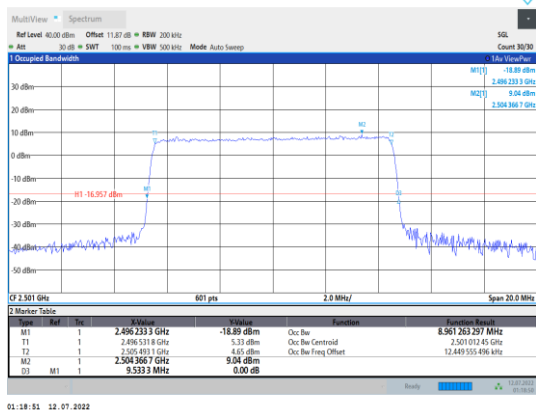
Band41-10MHz-QPSK-39700-50RB#0
