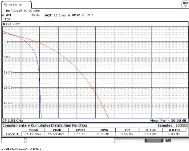
Band25-10MHz-QPSK-26640-1RB#0
