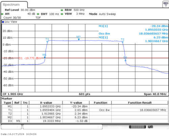
Band25-20MHz-QPSK-26590-100RB#0-18.037
