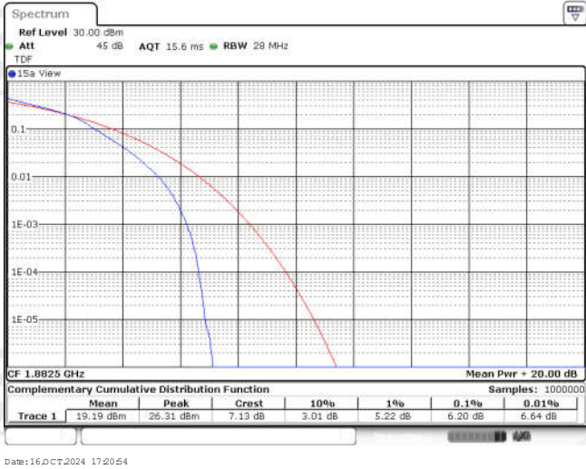
Band25-10MHz-16QAM-26365-25RB#0
