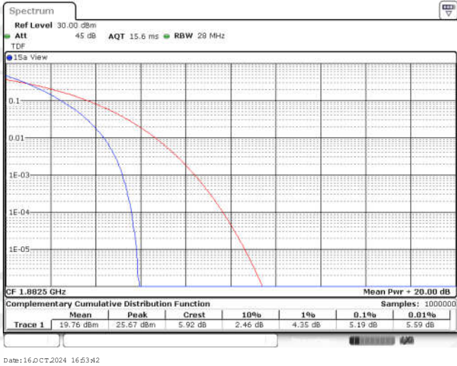
Band25-20MHz-QPSK-26365-100RB#0
