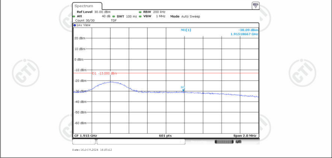
Band25-10MHz-QPSK-26640-1RB#0
