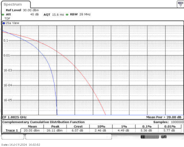
Band25-10MHz-QPSK-26365-50RB#0
