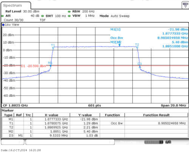
Band25-10MHz-QPSK-26365-50RB#0-8.985
