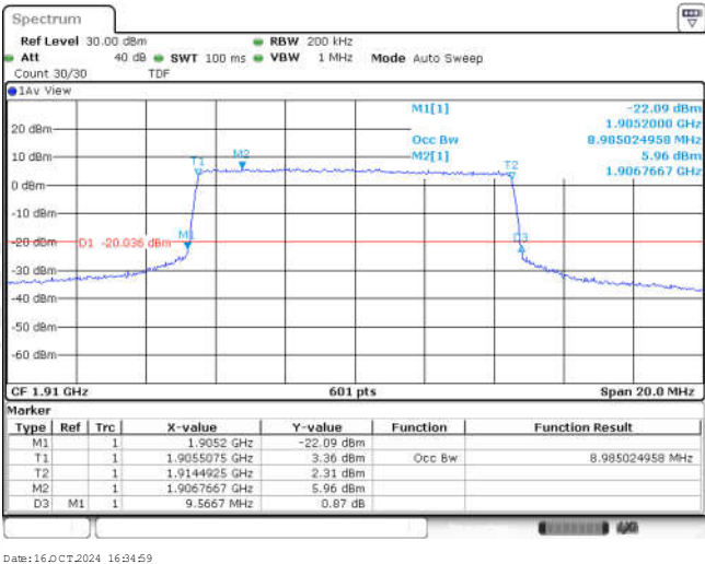
Band25-10MHz-QPSK-26640-50RB#0-8.985
