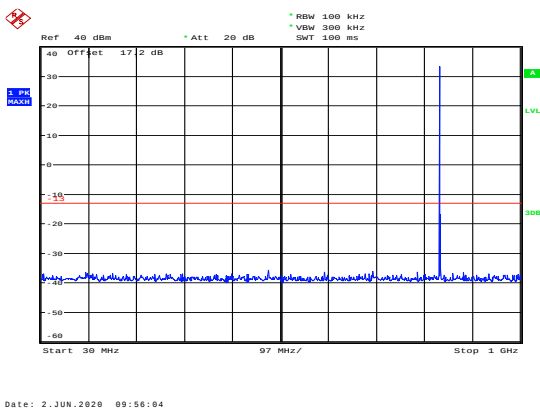
GSM 850 CH- Middle 30MHz ~ 1GHz
