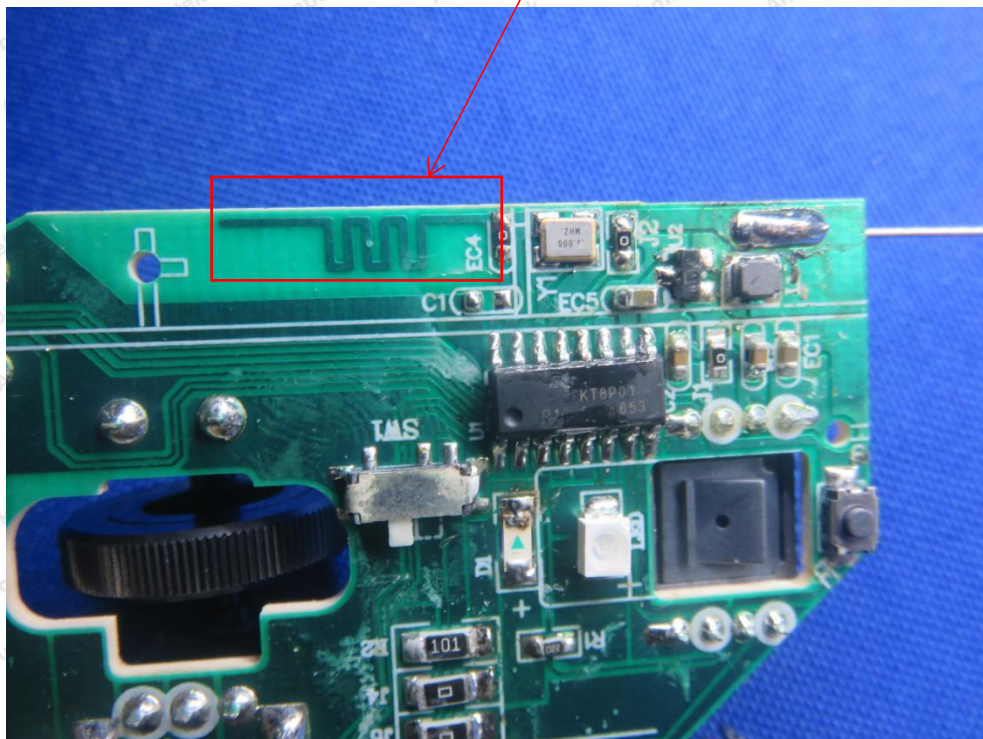
TX ANT
