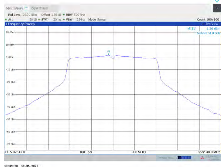
11a_Ant0_5825
