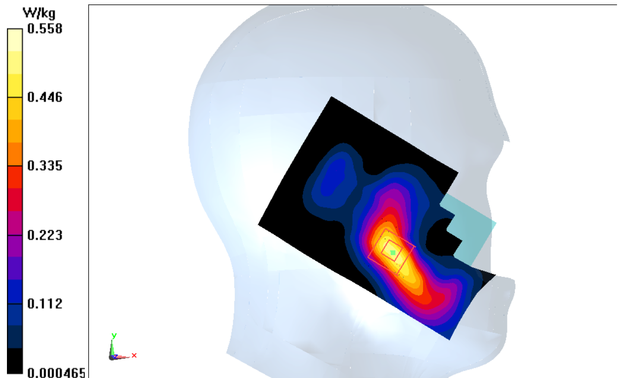
Fig.11 LTE Band7
