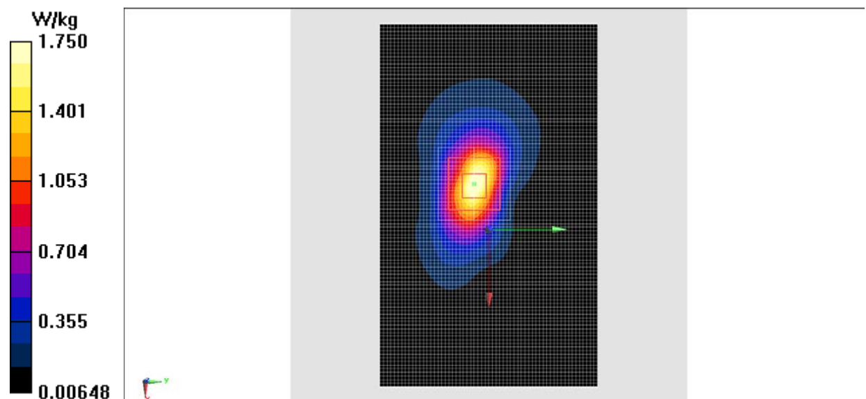
Fig.12 LTE Band7
