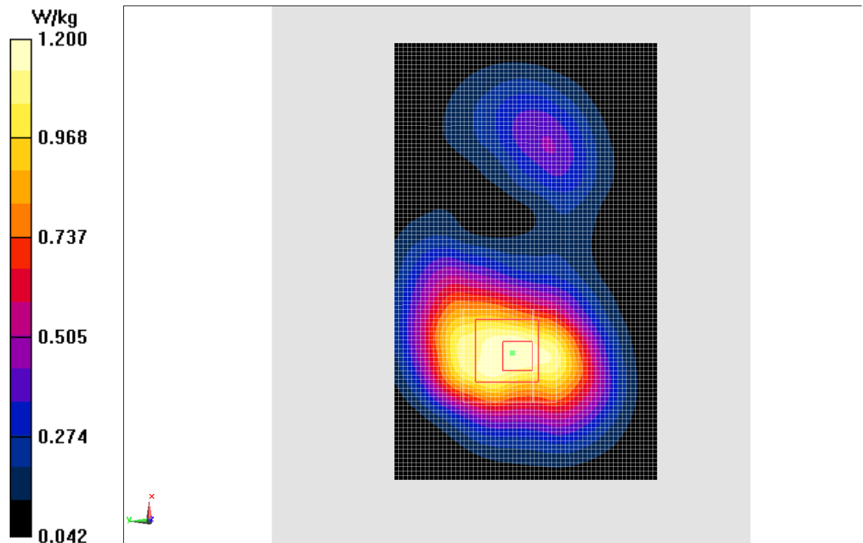
Fig.8 WCDMA1900
