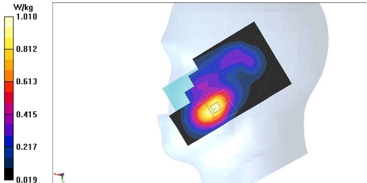
Fig.7 WCDMA1900
