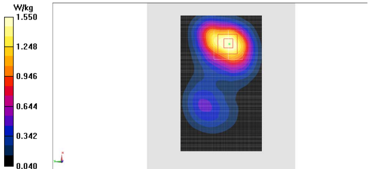
Fig.10 LTE Band4
