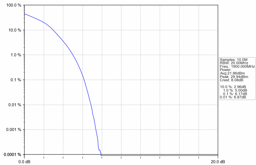
Band2 20MHz 16QAM HCH 1900MHz RB 100 0 NTN
