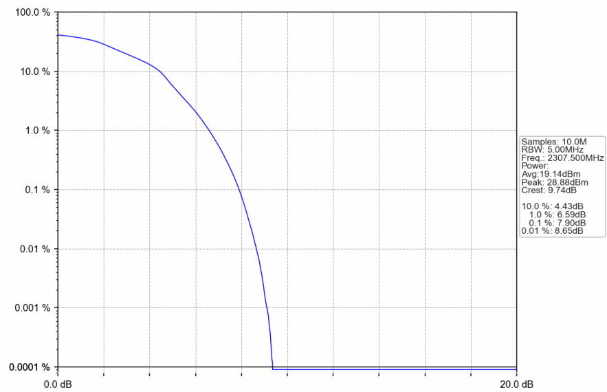
Band40a 5MHz 16QAM LCH 2307.5MHz RB 25 0 NTN
