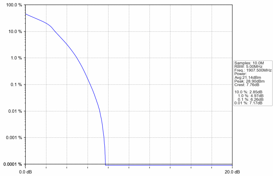
Band2 5MHz 16QAM HCH 1907.5MHz RB 25 0 NTNV
