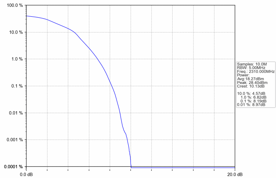
Band40a 5MHz 16QAM MCH 2310MHz RB 25 0 NTN
