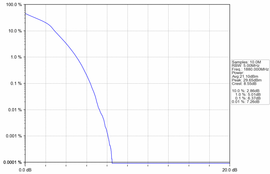
Band2 5MHz 16QAM MCH 1880MHz RB 25 0 NTNV
