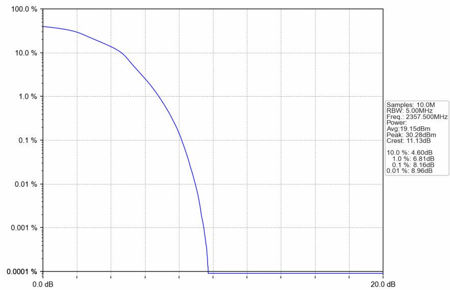
Band40b 5MHz 16QAM HCH 2357.5MHz RB 25 0 NTN
