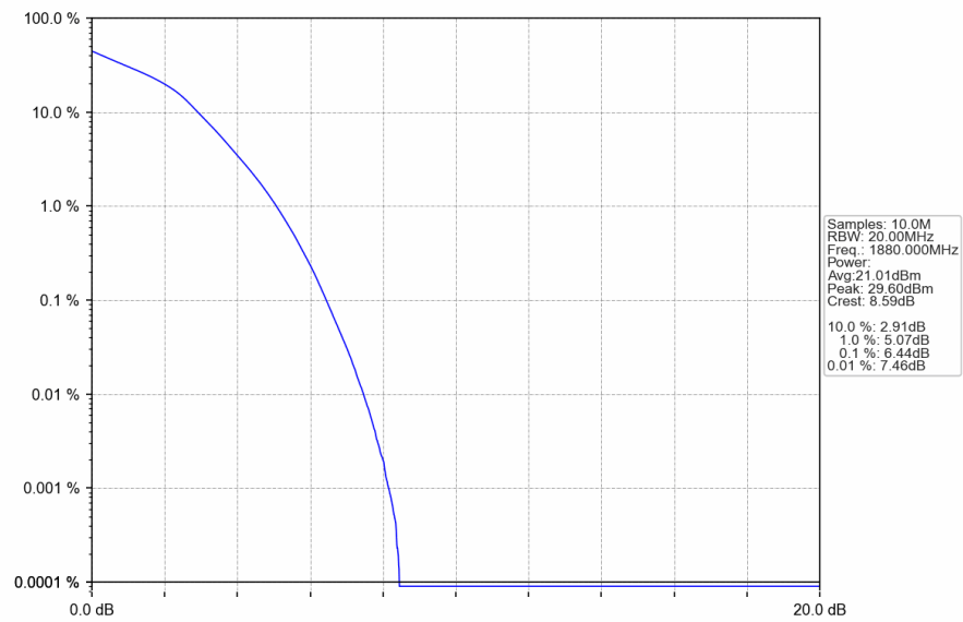
Band2 20MHz 16QAM MCH 1880MHz RB 100 0 NTN
