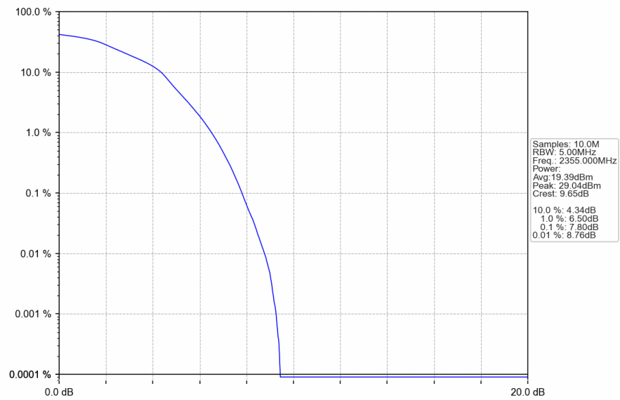
Band40b 5MHz 16QAM MCH 2355MHz RB 25 0 NTN
