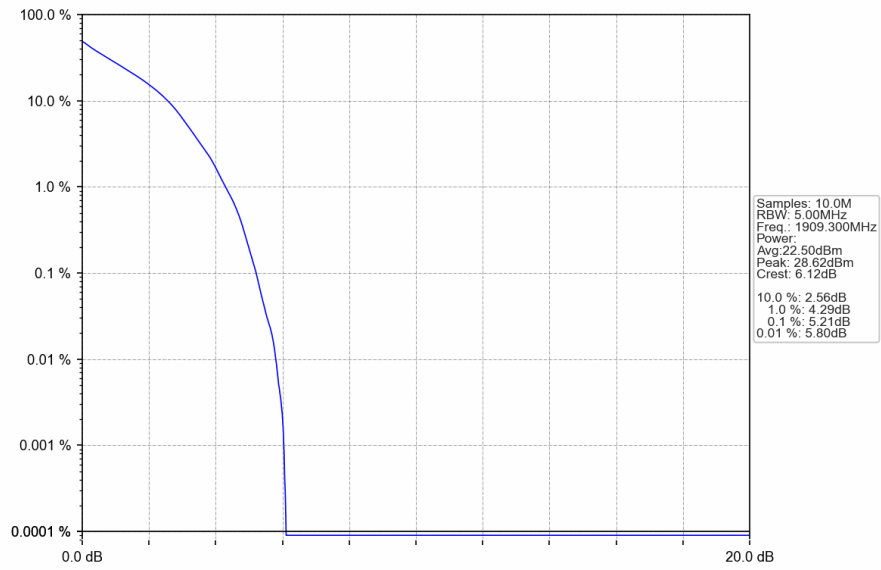
Band2 1.4MHz QPSK HCH 1909.3MHz RB 6 0 NTNV
