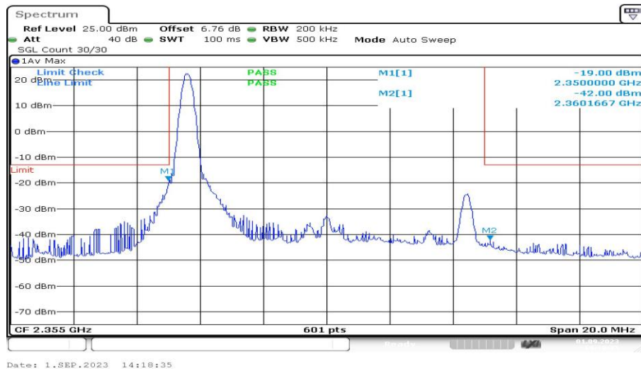
Band40-10MHz-QPSK-39200-1RB#0-PASS
