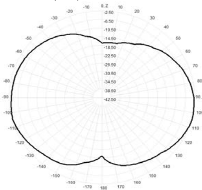
913.0MHz Total(E2-YZ), Max= -2.50dBi
