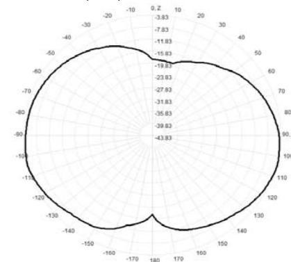
928.0MHz Total(E2-YZ), Max= -3.83dBi
