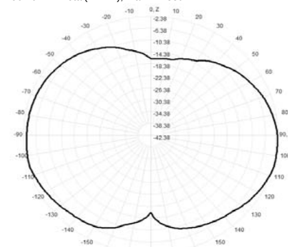
904.0MHz Total(E2-YZ), Max= -2.38dBi
