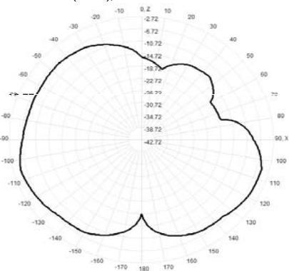
915.0MHz Total(E1-XZ), Max= -4.95dBi
