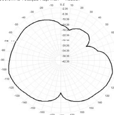
906.0MHz Total(E1-XZ), Max= -4.32dBi
