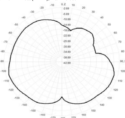
917.0MHz Total(E1-XZ), Max= -5.08dBi
