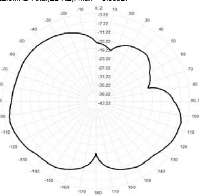
922.0MHz Total(E1-XZ), Max= -5.36dBi
