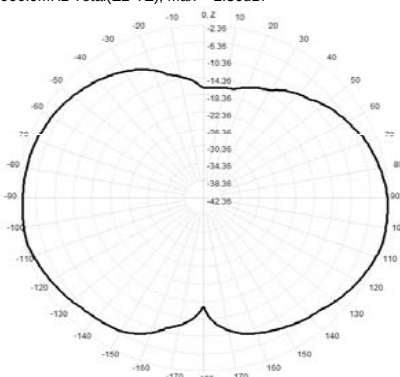
906.0MHz Total(E2-YZ), Max= -2.36dBi
