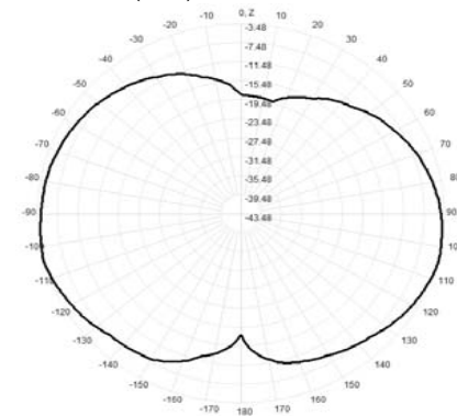
925.0MHz Total(E2-YZ), Max= -3.48dBi
