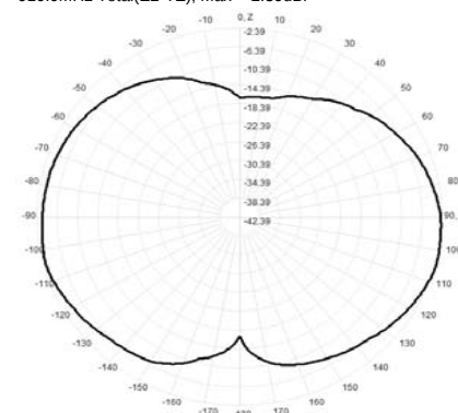
910.0MHz Total(E2-YZ), Max= -2.39dBi
