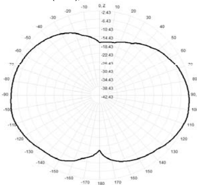
912.0MHz Total(E2-YZ), Max= -2.43dBi
