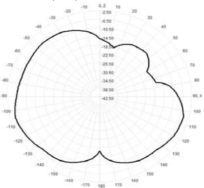
913.0MHz Total(E1-XZ), Max= -4.75dBi
