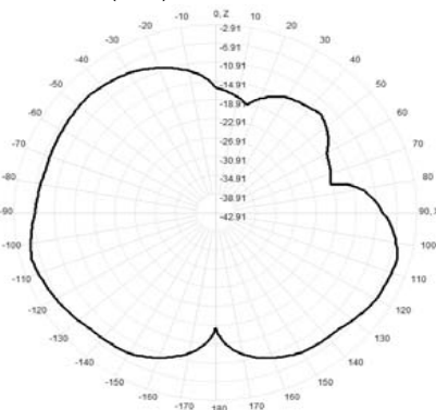
919.0MHz Total(E1-XZ), Max= -5.16dBi
