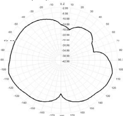
918.0MHz Total(E1-XZ), Max= -5.14dBi
