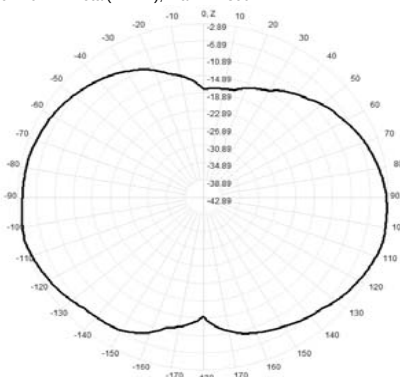
917.0MHz Total(E2-YZ), Max= -2.89dBi
