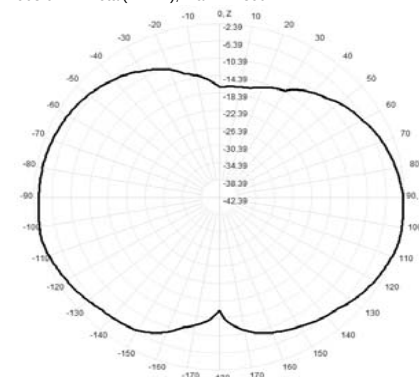
908.0MHz Total(E2-YZ), Max= -2.39dBi
