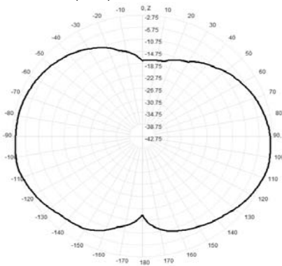
916.0MHz Total(E2-YZ), Max= -2.75dBi
