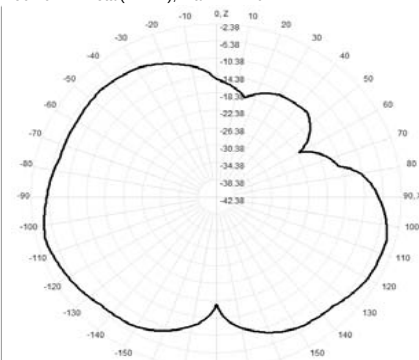
904.0MHz Total(E1-XZ), Max= -4.27dBi
