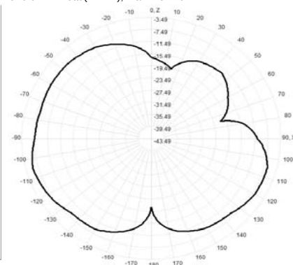
926.0MHz Total(E1-XZ), Max= -5.72dBi
