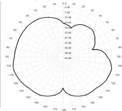
925.0MHz Total(E1-XZ), Max= -5.57dBi
