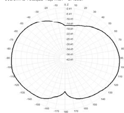
904.0MHz Total(E2-YZ), Max= -2.38dBi
