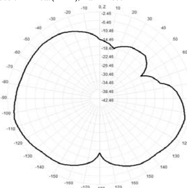
905.0MHz Total(E1-XZ), Max= -4.35dBi
