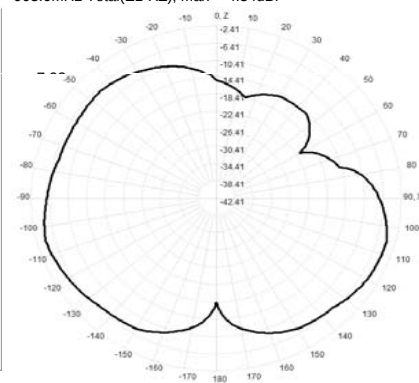
904.0MHz Total(E1-XZ), Max= -4.27dBi
