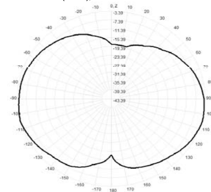
924.0MHz Total(E2-YZ), Max= -3.39dBi
