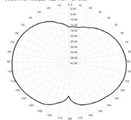
903.0MHz Total(E2-YZ), Max= -2.41dBi
