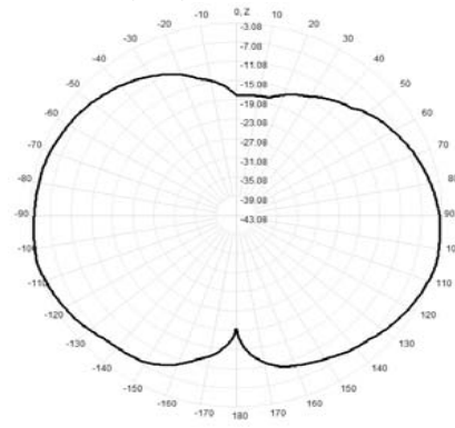
921.0MHz Total(E2-YZ), Max= -3.24dBi
