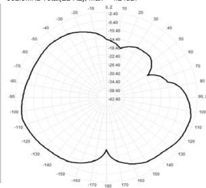
903.0MHz Total(E1-XZ), Max= -4.34dBi
