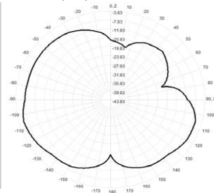
928.0MHz Total(E1-XZ), Max= -5.95dBi
