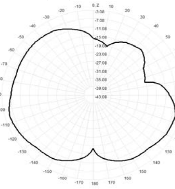
921.0MHz Total(E1-XZ), Max= -5.30dBi
