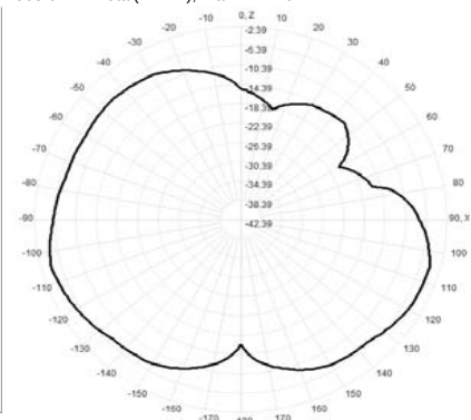
908.0MHz Total(E1-XZ), Max= -4.41dBi
