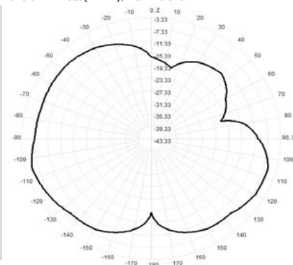
923.0MHz Total(E1-XZ), Max= -5.34dBi
