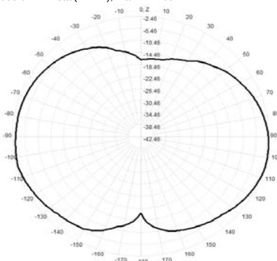
905.0MHz Total(E2-YZ), Max= -2.46dBi
