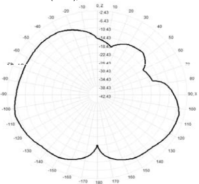
912.0MHz Total(E1-XZ), Max= -4.74dBi
