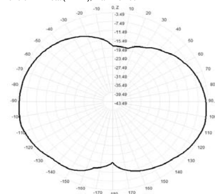
926.0MHz Total(E2-YZ), Max= -3.49dBi
