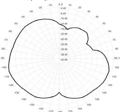
911.0MHz Total(E1-XZ), Max= -4.62dBi
