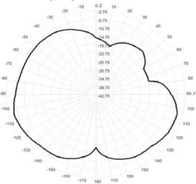
916.0MHz Total(E1-XZ), Max= -5.08dBi
