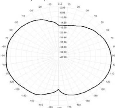
918.0MHz Total(E2-YZ), Max= -2.98dBi
