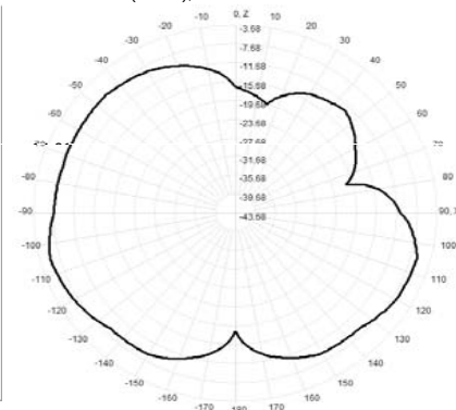
927.0MHz Total(E1-XZ), Max= -5.72dBi
