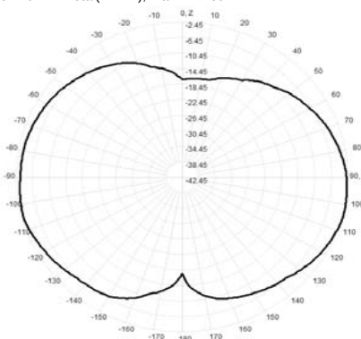
911.0MHz Total(E2-YZ), Max= -2.45dBi
