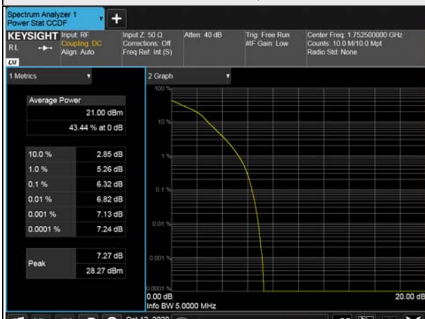
15MHz / 16QAM
