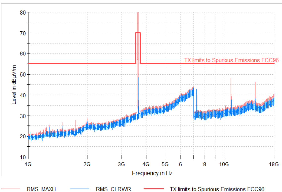
RF_FCC_Part96_E Field_1GHz_18GHz
