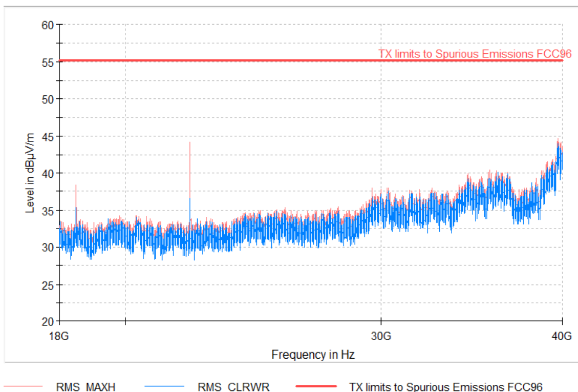
RF_FCC_Part96_E Field_18GHz_40GHz
