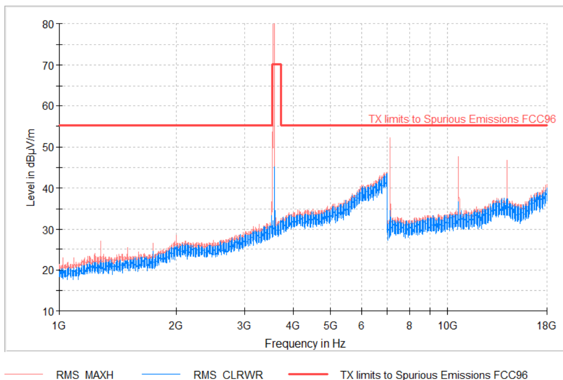
RF_FCC_Part96_E Field_1GHz_18GHz
