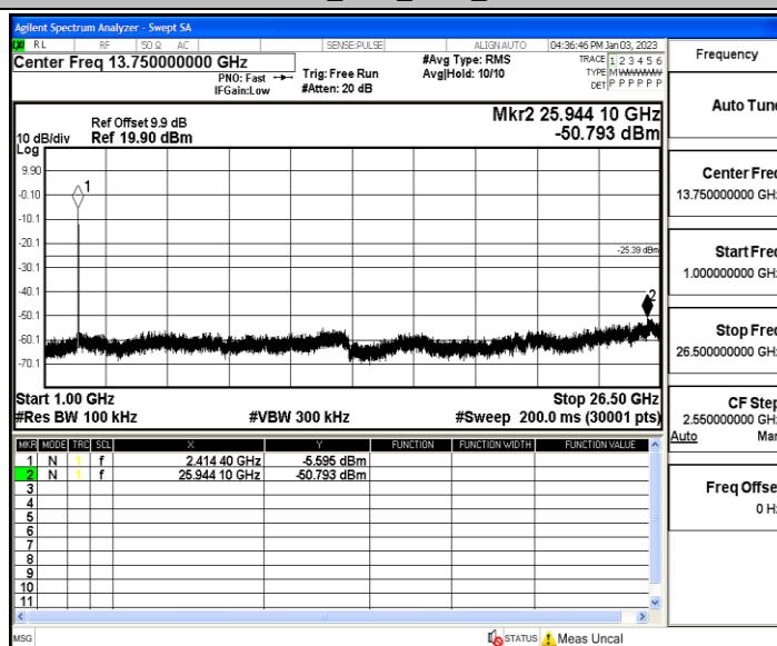
11AX20MIMO_Ant2_2412_0~Reference
