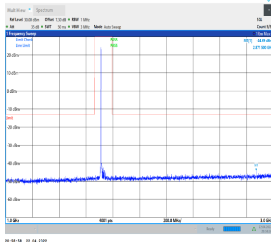
1-N66-PC3-15-40-L-1-DFT-PI2BPSK-Inner_1RB_Lef t-1@1-1000-3000-Ant0--44.39--13-PASS
