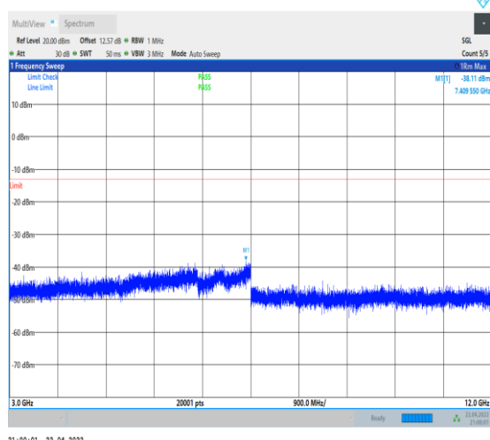
1-N66-PC3-15-40-M-1-DFT-PI2BPSK-Inner_1RB_L eft-1@1-3000-12000-Ant0--38.11--13-PASS
