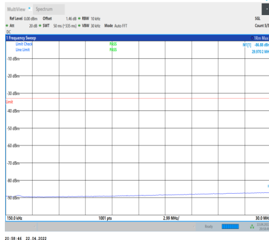
1-N66-PC3-15-40-L-1-DFT-PI2BPSK-Inner_1RB_Lef t-1@1-0.15-30-Ant0--86.88--33-PASS
