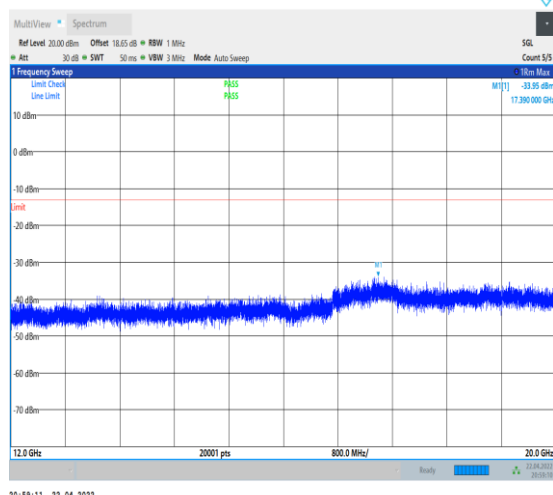
1-N66-PC3-15-40-L-1-DFT-PI2BPSK-Inner_1RB_Lef t-1@1-12000-20000-Ant0--33.95--13-PASS
