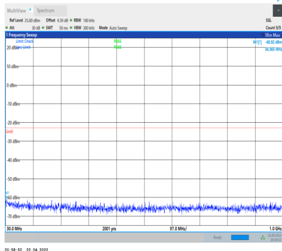
1-N66-PC3-15-40-L-1-DFT-PI2BPSK-Inner_1RB_Le ft-1@1-30-1000-Ant0--60.92--23-PASS
