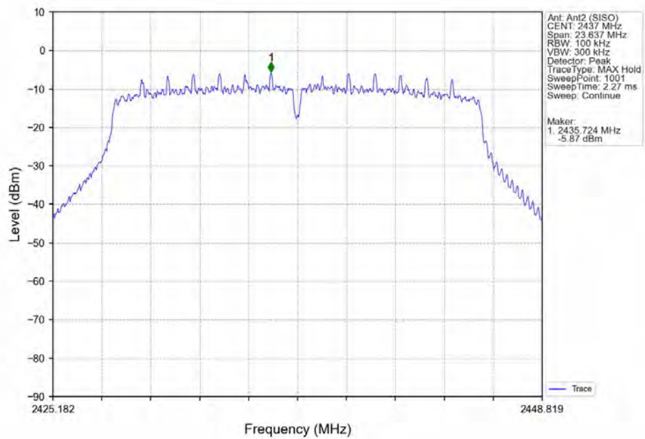
802.11ax(HEW20)_MCH_2437MHz_Ant2 (SISO)_NTNV
