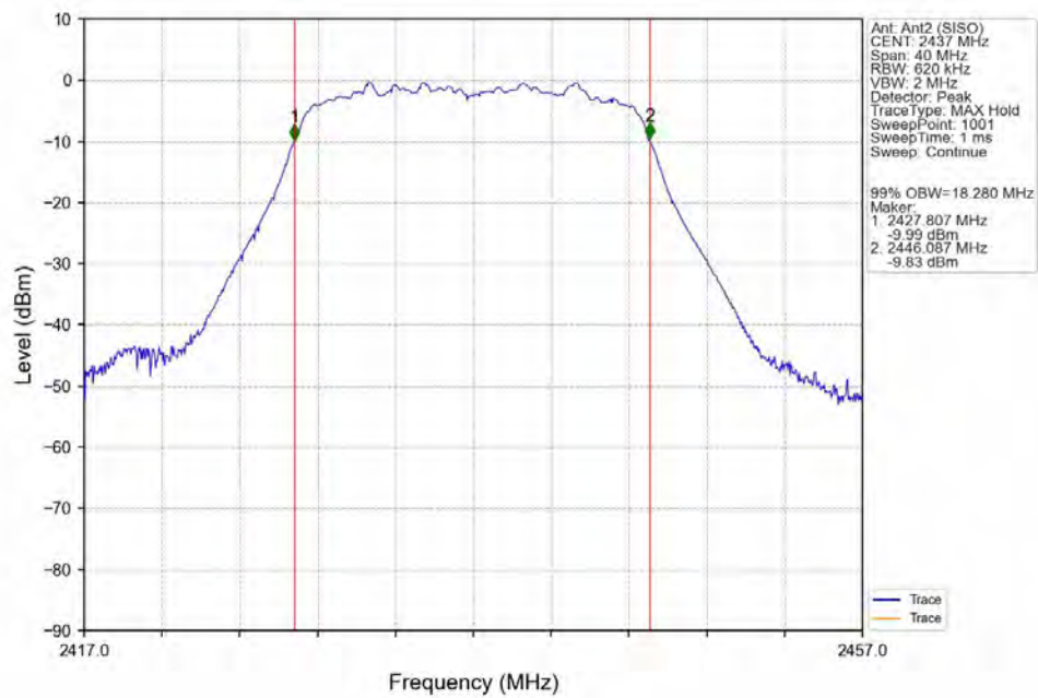
802.11ax(HEW20)_MCH_2437MHz_Ant2 (SISO)_NTNV
