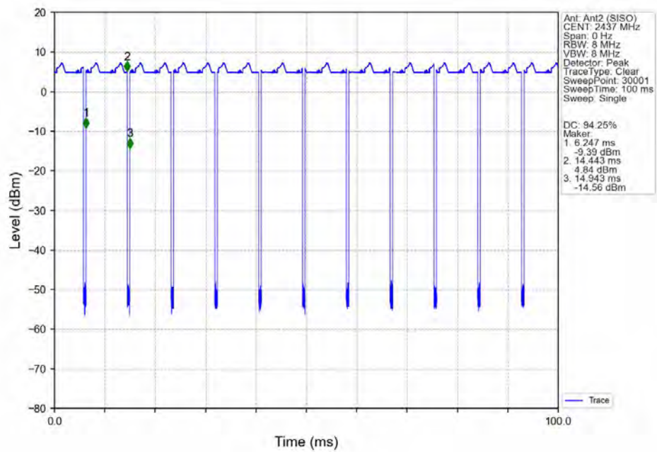
802.11b_MCH_2437MHz_Ant2 (SISO)_NTNV
