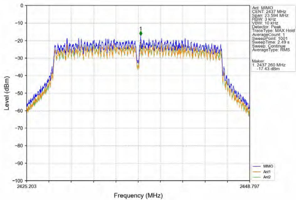
802.11ax(HEW20)_MCH_2437MHz_MIMO_NTNV
