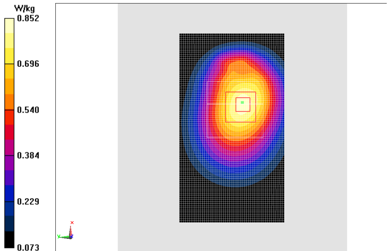
Fig.6 WCDMA 850 CH4182
