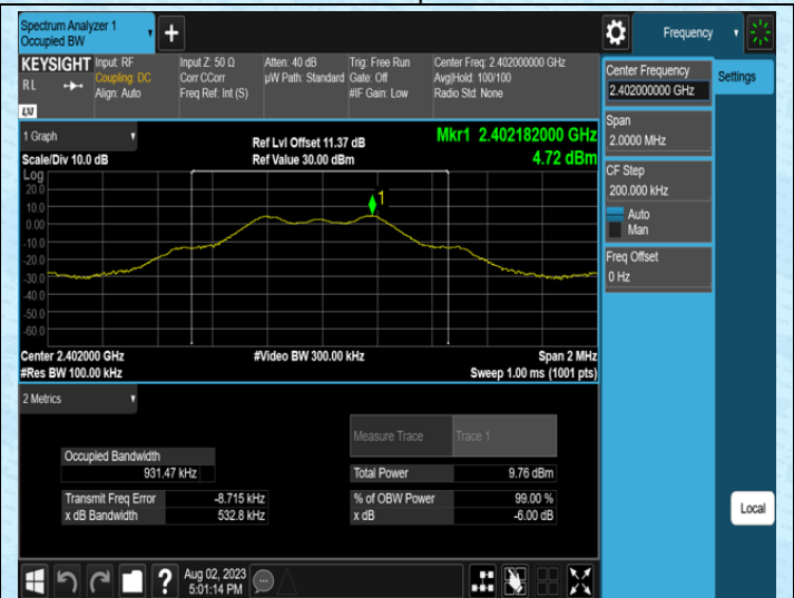
TX-Ant2-2402
