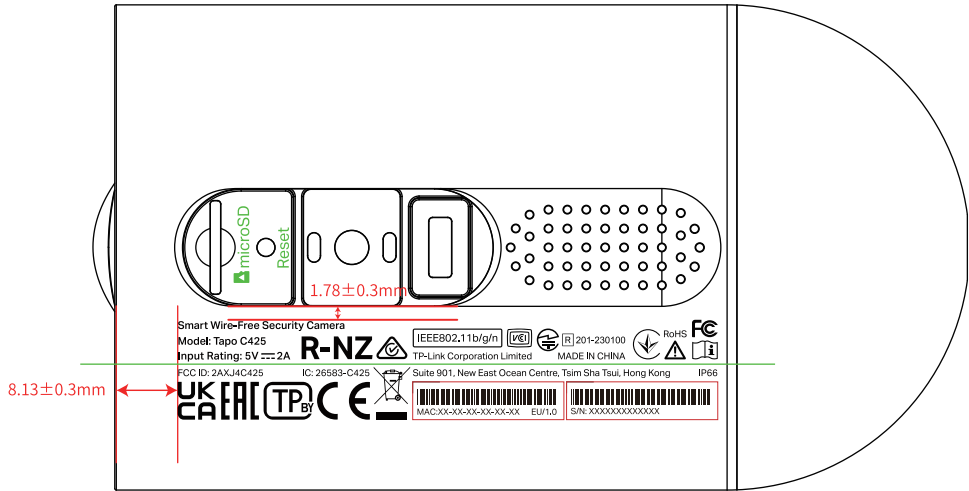
尺寸图
