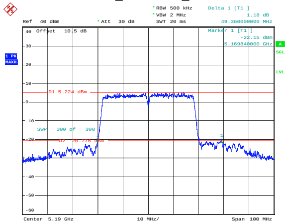
802.11n40_5190MHz_Chain 0
