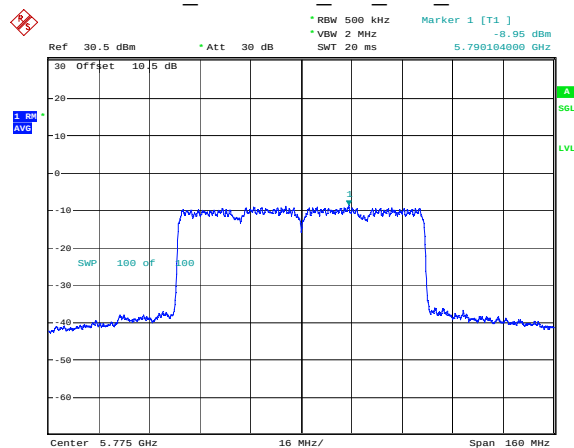
802.11ax80 5775MHz RU Full Chain 1
