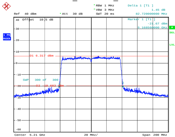
802.11ac80_5210MHz_Chain 0
