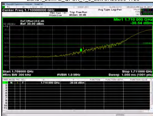
Band4_20MHz_QPSK_1_0_LowCH20050-1720
