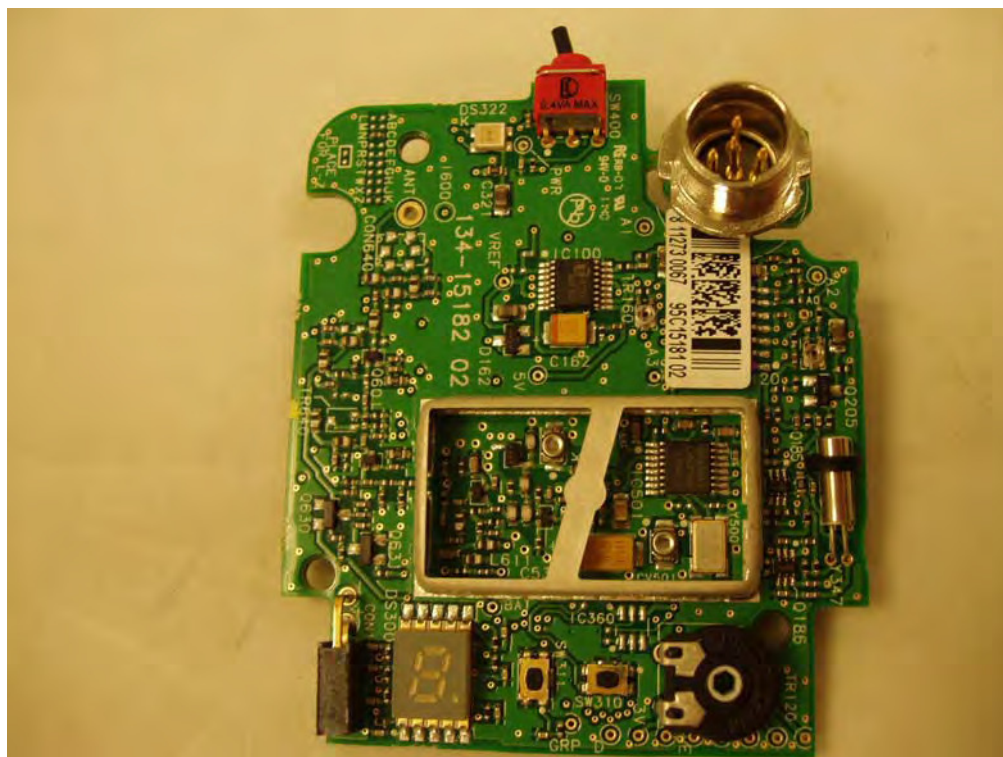
BLX1 PCB Top
