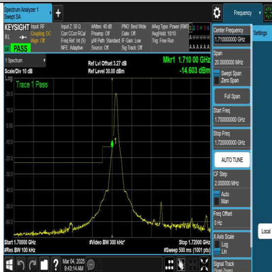
NTVN-N66-PC3-15-10-L-DFT-QPSK-Edge_1RB_Left-Ant1-PASS
