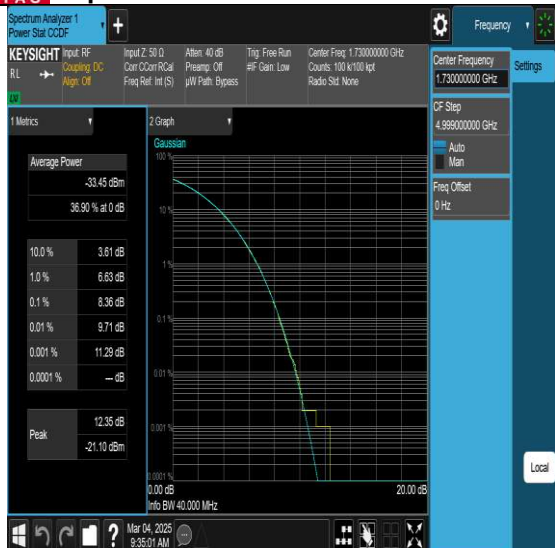
NTNV-N66-PC3-15-40-L-DFT-QPSK-Edge 1RB Left-PASS
