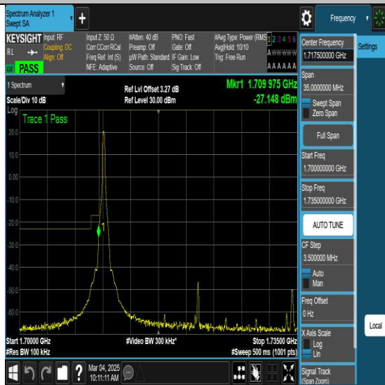
NTNV-N66-PC3-15-25-L-DFT-QPSK-Edge_1RB_Left-Ant1-
