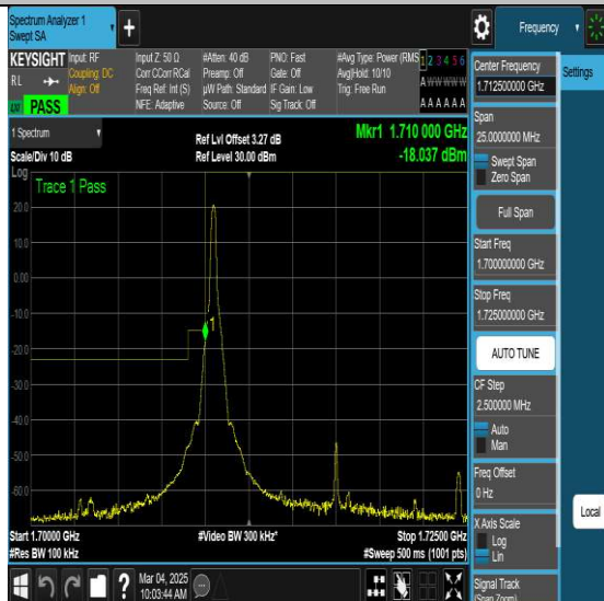
NTNV-N66-PC3-15-15-L-DFT-QPSK-Edge_1RB_Left-Ant1-PASS
