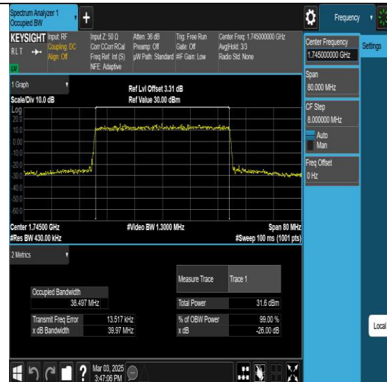
NTNV-N66-PC3-15-40-M-DFT-QPSK-Outet_Full-Ant1-PASS
