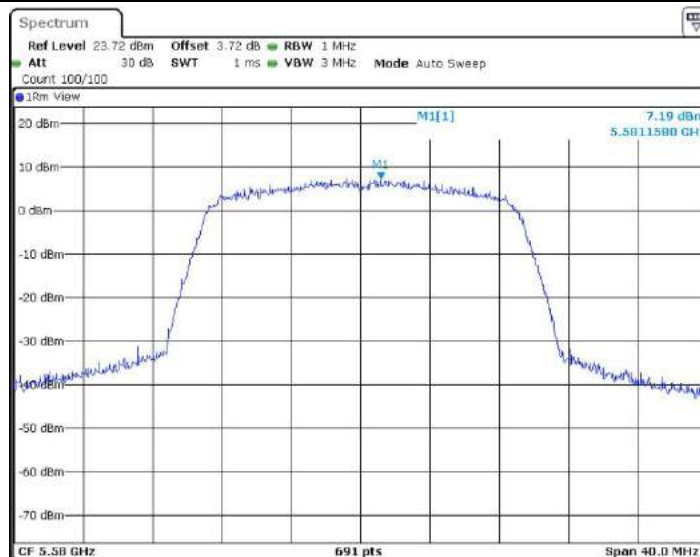
11AC20MIMO_Ant1_5580
