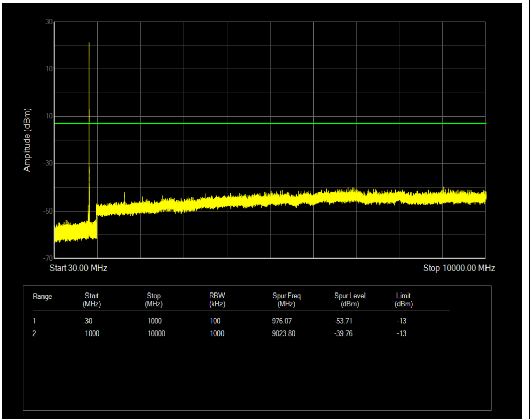
n26(824-849) SCS=15kHz DFT_BPSK BW=20MHz Channel=166800 RB=1@0
