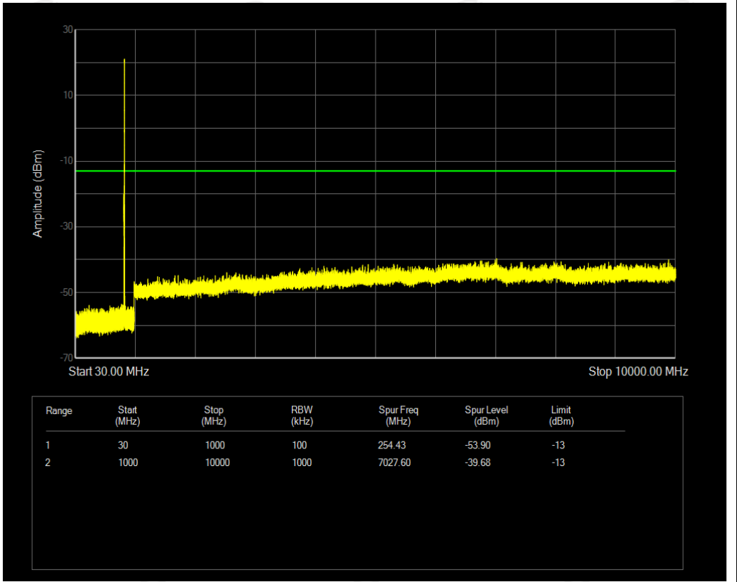
n26(824-849) SCS=15kHz DFT_BPSK BW=10MHz Channel=167300 RB=1@51
