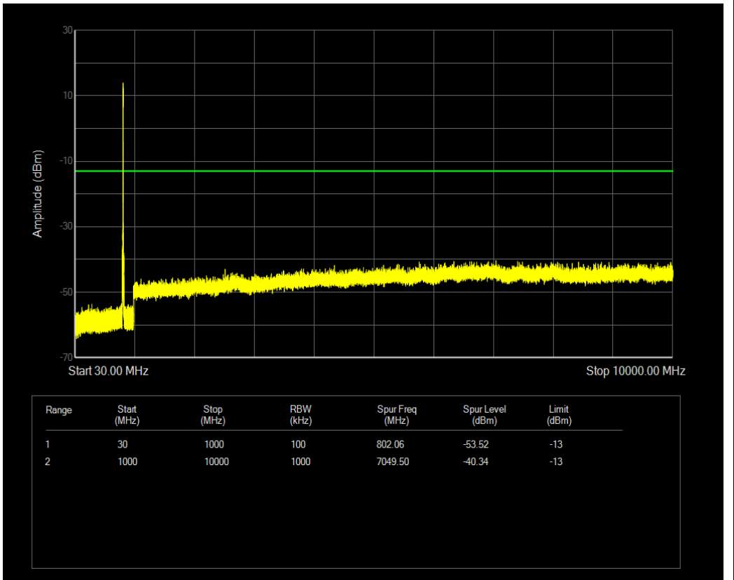
n26(824-849) SCS=15kHz DFT_BPSK BW=5MHz Channel=165300 RB=25@0
