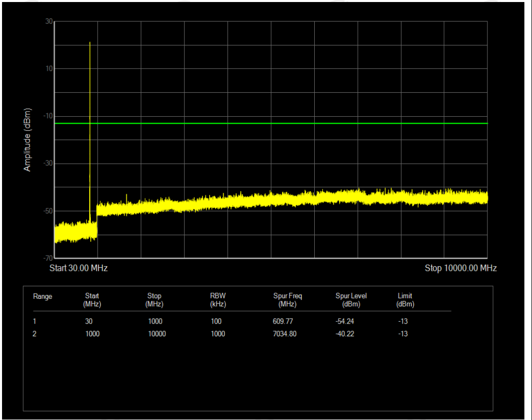
n26(824-849) SCS=15kHz DFT_BPSK BW=20MHz Channel=166800 RB=1@105
