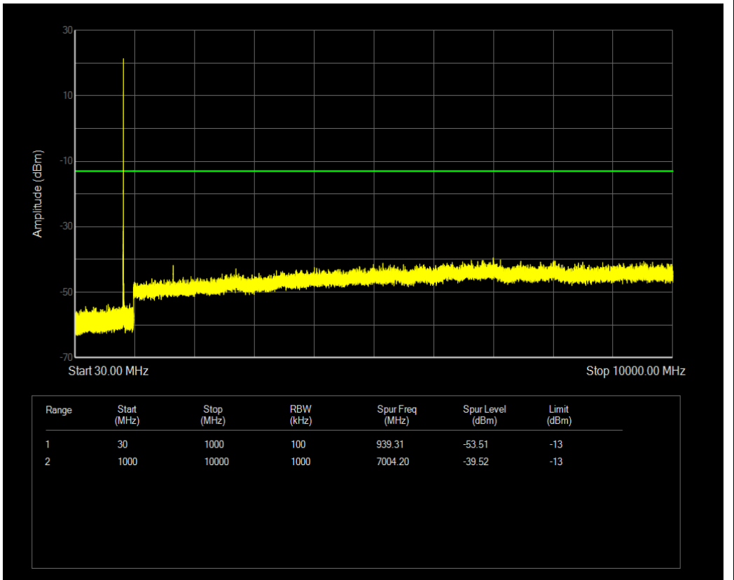
n26(824-849) SCS=15kHz DFT_BPSK BW=10MHz Channel=167300 RB=1@0
