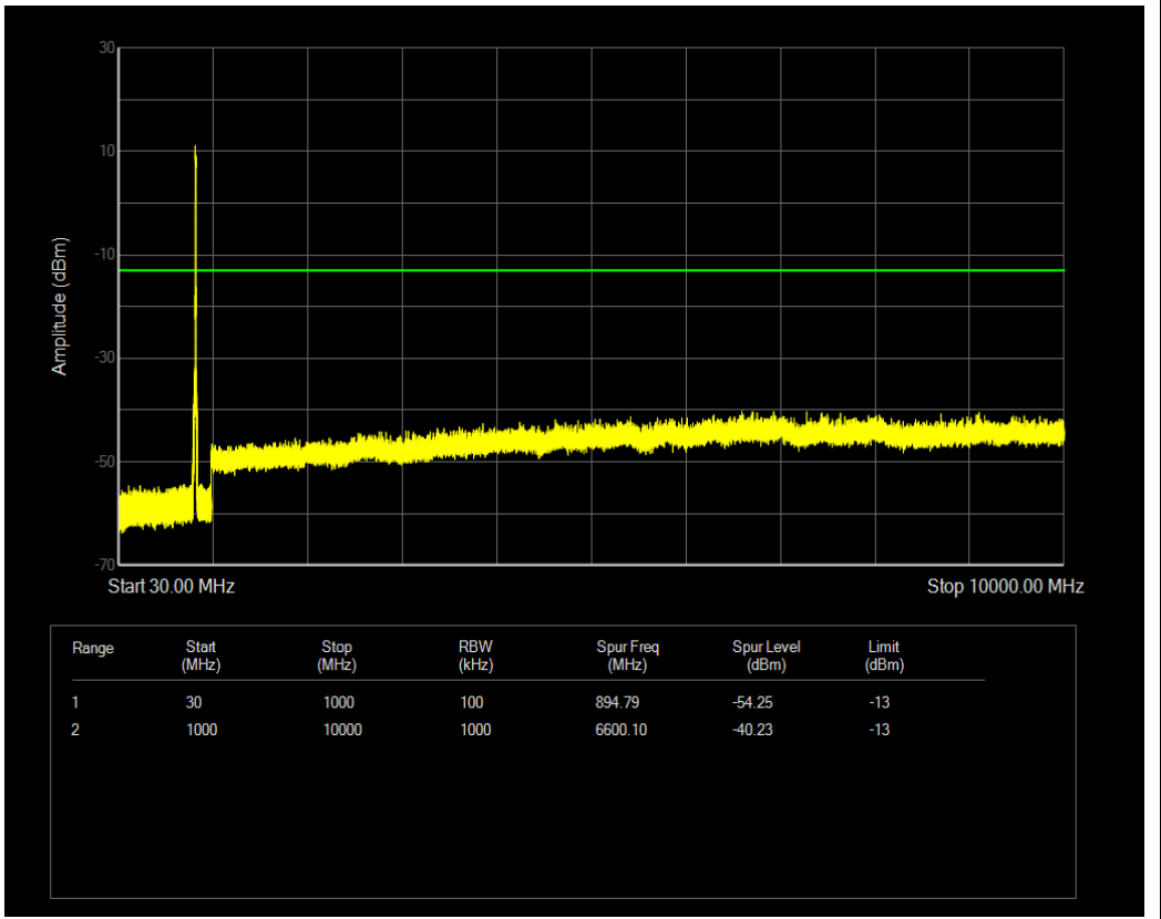
n26(824-849) SCS=15kHz DFT_BPSK BW=10MHz Channel=167300 RB=50@0
