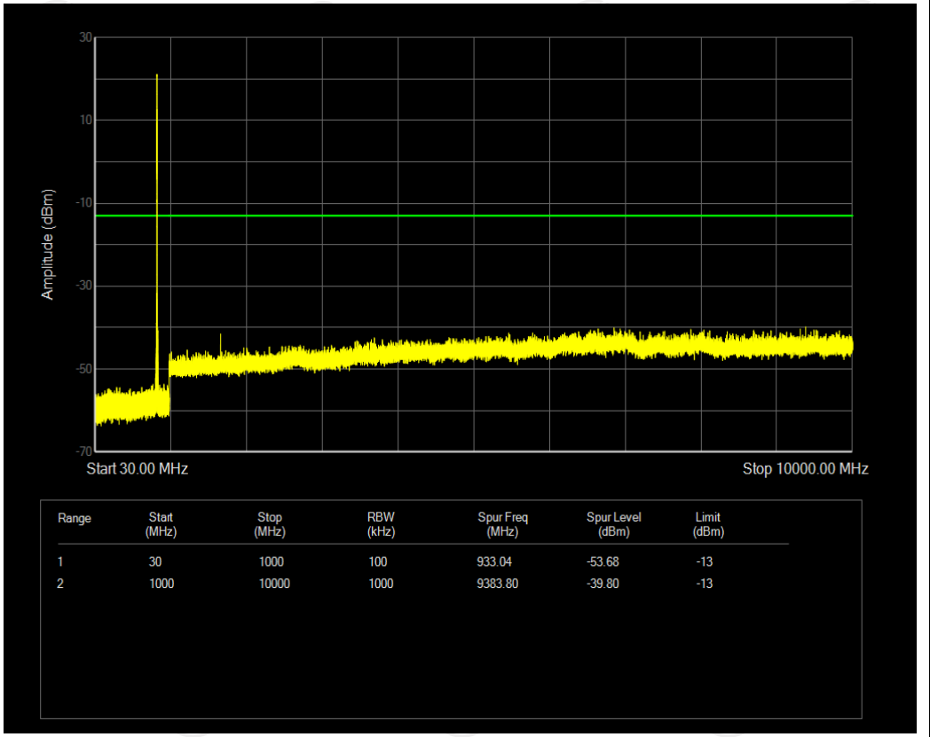
n26(824-849) SCS=15kHz DFT_BPSK BW=10MHz Channel=168800 RB=1@0
