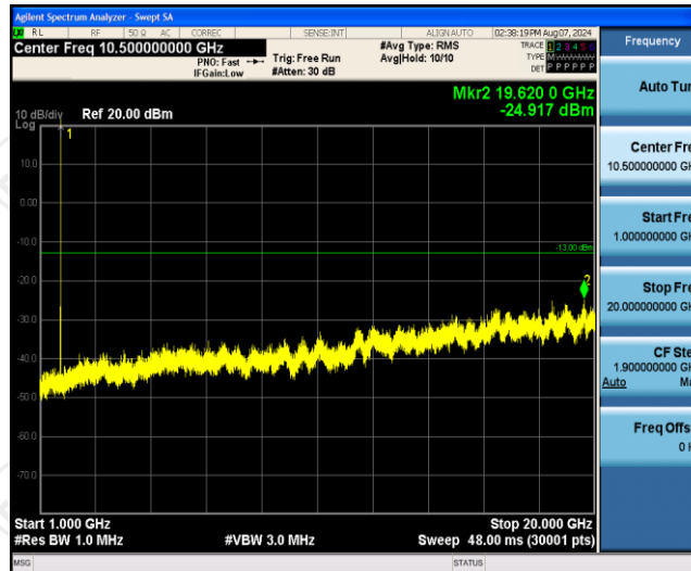
Band66-3MHz-QPSK-131987-1RB#0-Range2:1000~20000MHz
