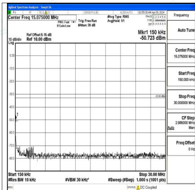
Band4 15MHz 16QAM 20175 1RB#0 0.15~30 0.15~30
