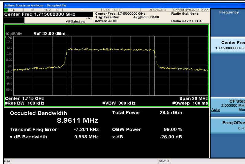
Band4-10MHz-QPSK-20000-50RB#0-8.9611
