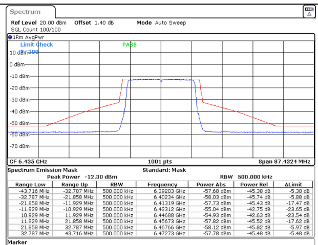
802.11ax (20MHz) 6435MHz Chain B NSS-2
