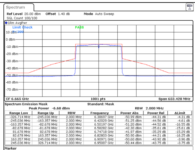
802.11ax (160MHz) 6665MHz Chain D NSS-1
