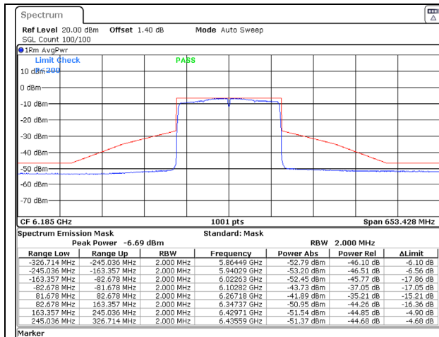
802.11ax (160MHz) 6185MHz Chain C NSS-1
