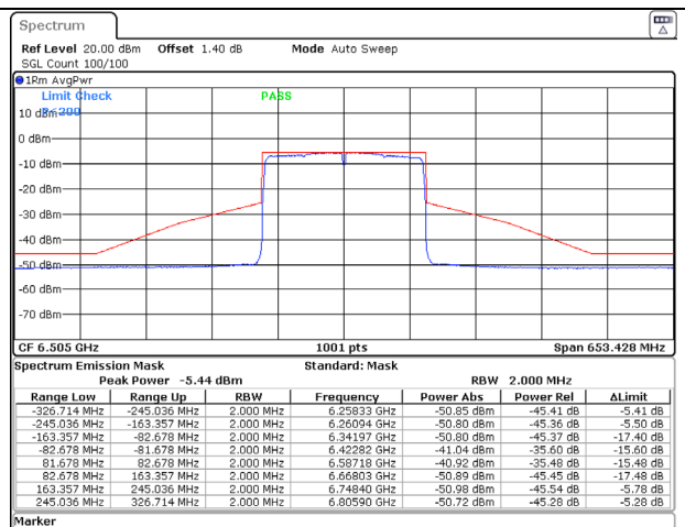
802.11ax (160MHz) 6505MHz Chain B NSS-1
