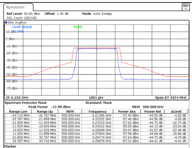
802.11ax (20MHz) 6255MHz Chain D NSS-2
