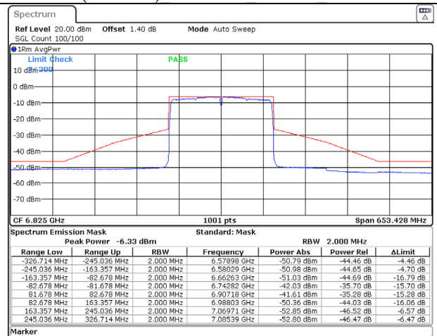
802.11ax (160MHz) 6825MHz Chain D NSS-1
