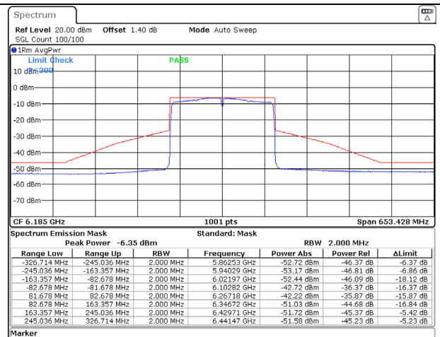
802.11ax (160MHz) 6185MHz Chain D NSS-1
