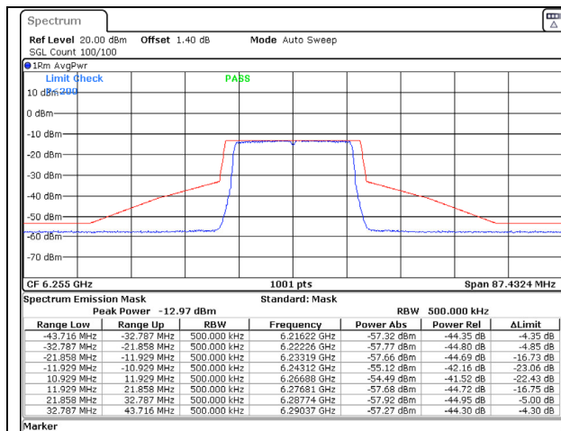
802.11ax (20MHz) 6255MHz Chain C NSS-2
