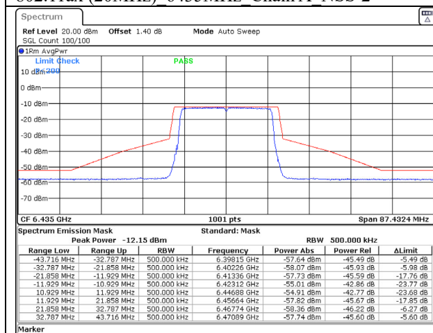
802.11ax (20MHz) 6435MHz Chain C NSS-2
