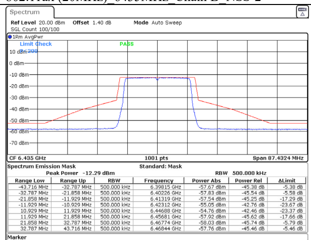
802.11ax (20MHz) 6435MHz Chain D NSS-2
