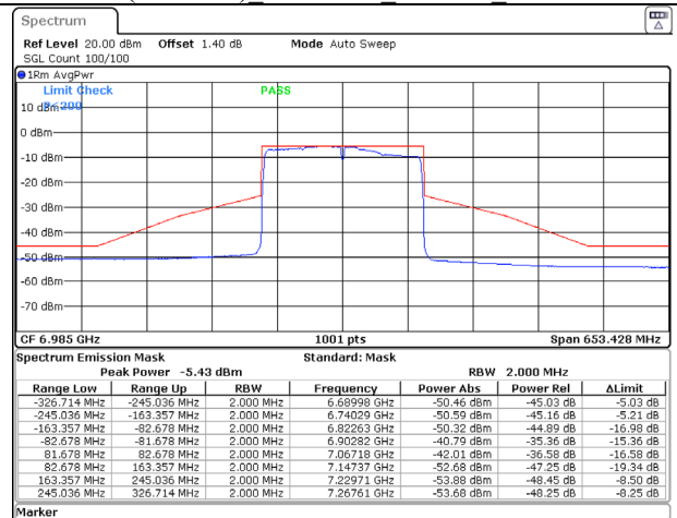
802.11ax (160MHz) 6985MHz Chain D NSS-1
