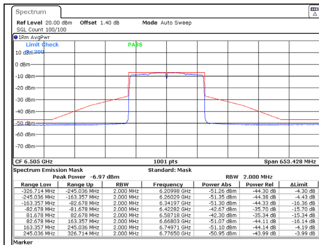
802.11ax (160MHz) 6505MHz Chain A NSS-1
