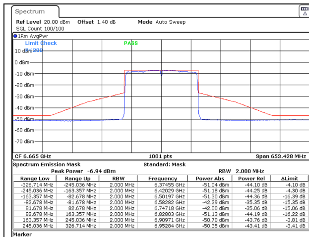
802.11ax (160MHz) 6665MHz Chain C NSS-1
