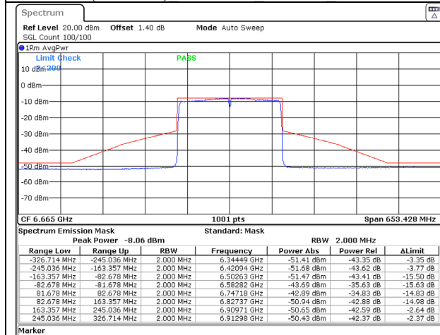
802.11ax (160MHz) 6665MHz Chain A NSS-1
