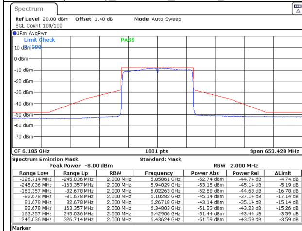
802.11ax (160MHz) 6185MHz Chain A NSS-1
