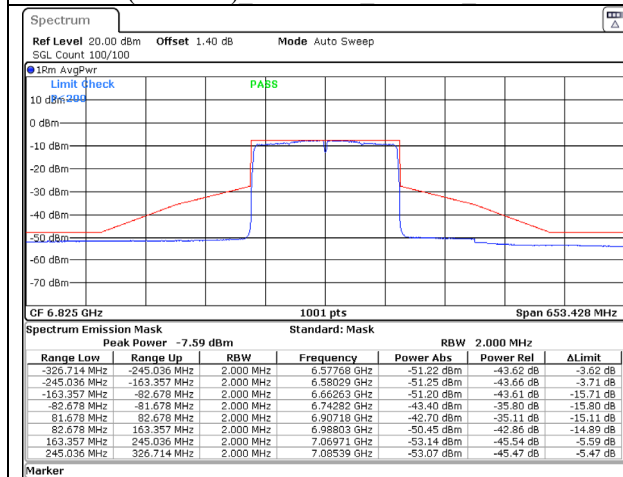
802.11ax (160MHz) 6825MHz Chain C NSS-1
