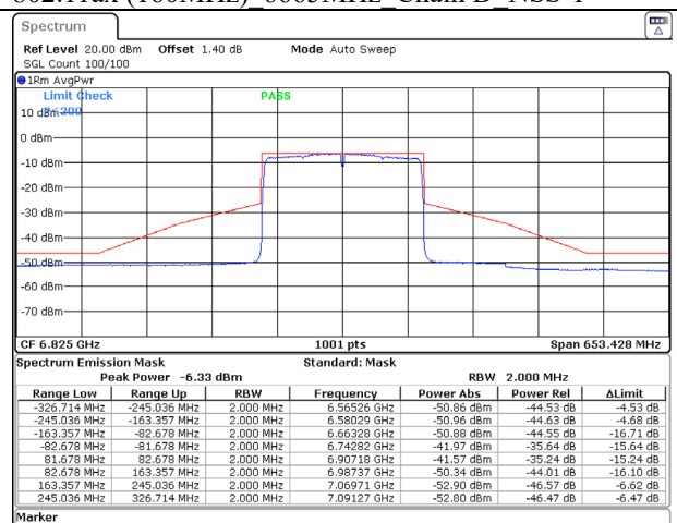
802.11ax (160MHz) 6825MHz Chain B NSS-1
