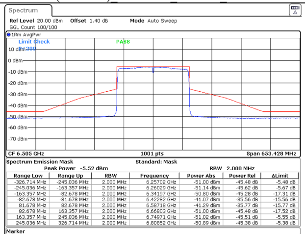
802.11ax (160MHz) 6505MHz Chain D NSS-1
