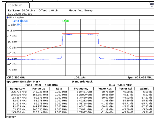
802.11ax (160MHz) 6505MHz Chain C NSS-1
