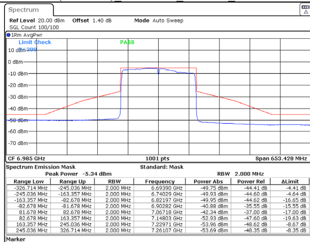
802.11ax (160MHz) 6985MHz Chain C NSS-1
