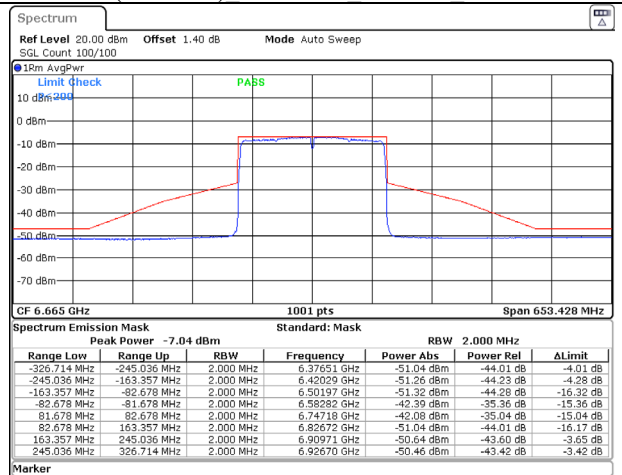
802.11ax (160MHz) 6665MHz Chain B NSS-1
