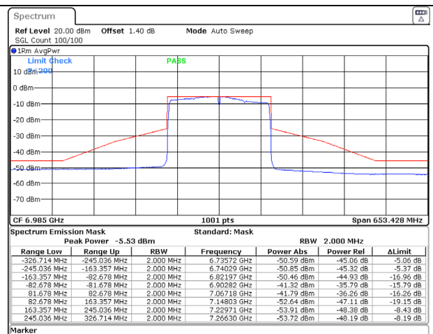
802.11ax (160MHz) 6985MHz Chain B NSS-1
