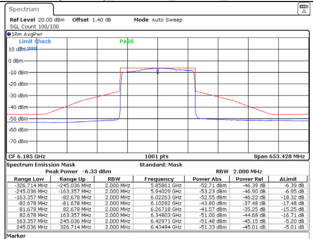
802.11ax (160MHz) 6185MHz Chain B NSS-1
