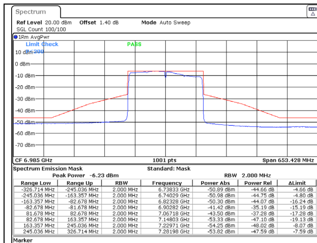
802.11ax (160MHz) 6985MHz Chain A NSS-1
