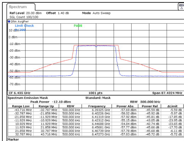
802.11ax (20MHz) 6435MHz Chain A NSS-2
