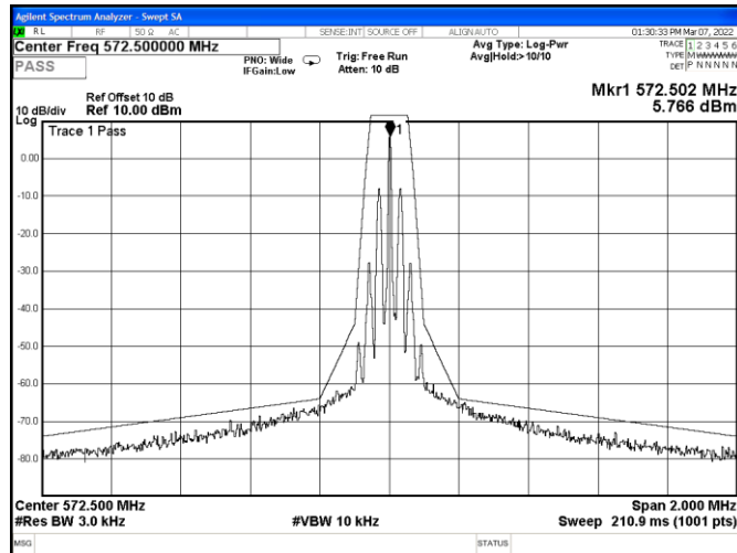
Channel 0/ 572.5 MHz
