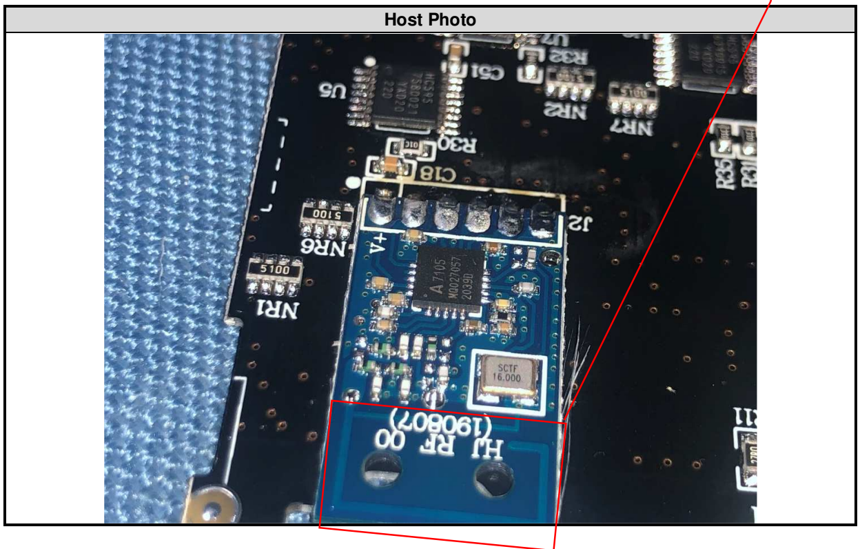
Antenna
