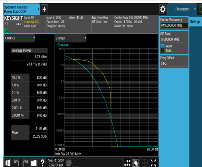
Band26-1.4MHz-QPSK-26740-1-0-Low-9.85-&lt;=13-PASS
