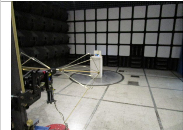
30-200 MHz
