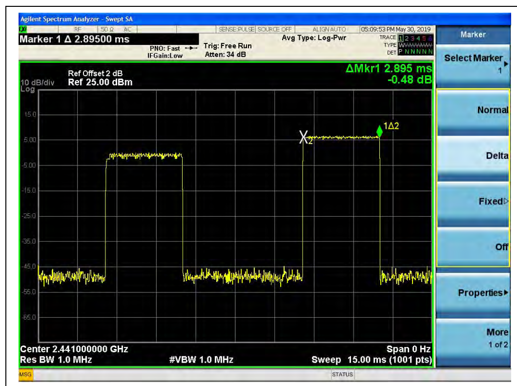
(DH5, 8-DPSK)
