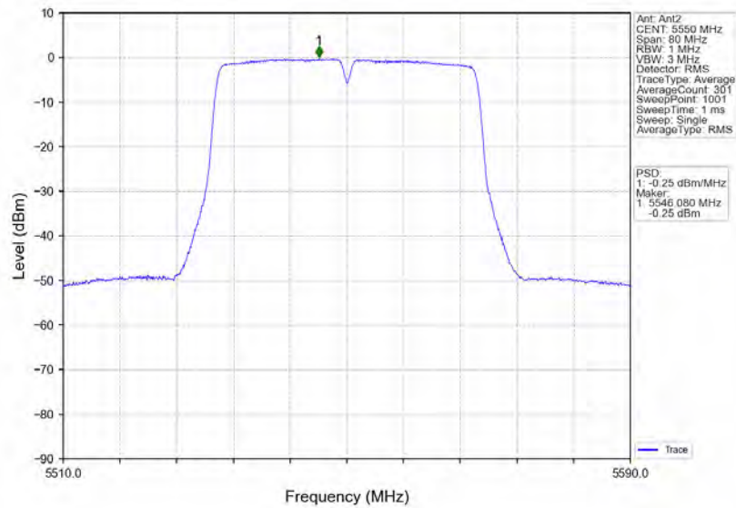
802.11n(HT40)_MCH_5550MHz_MIMO_NTNV
