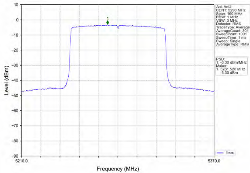
802.11ax(HEW80)_MCH_5290MHz_RU996_Left_Ant2_NTNV
