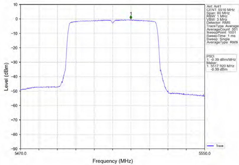
802.11ax(HEW40)_LCH_5510MHz_RU484_Left_Ant1_NTNV
