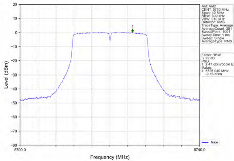
802.11a_HCH_5720MHz_Ant2_NTNV
