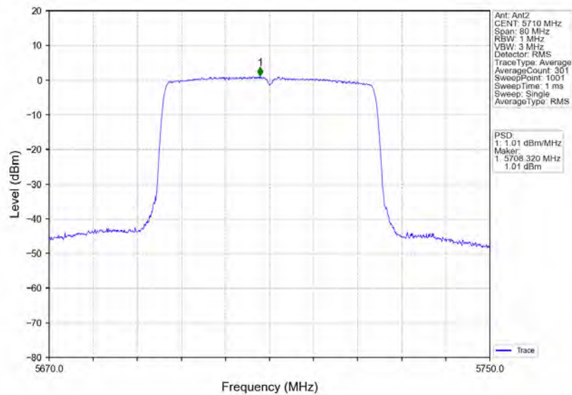
802.11ax(HEW40)_HCH_5710MHz_RU484_Left_Ant2_NTNV
