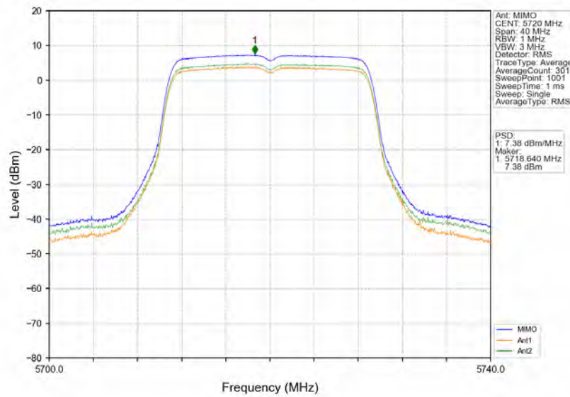
802.11n(HT20)_HCH_5720MHz_MIMO_NTNV
