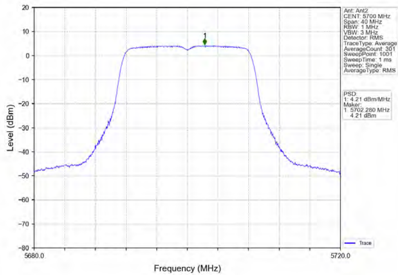
802.11a_HCH_5700MHz_Ant2_NTNV
