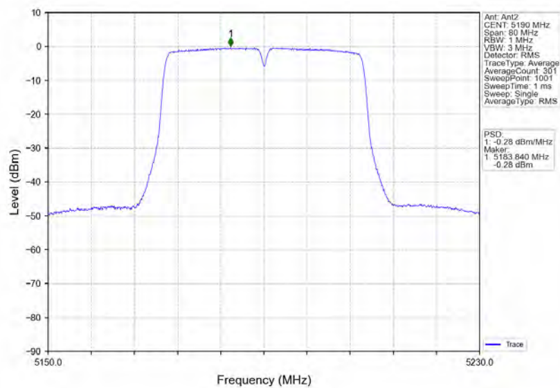
802.11n(HT40)_LCH_5190MHz_Ant2_NTNV
