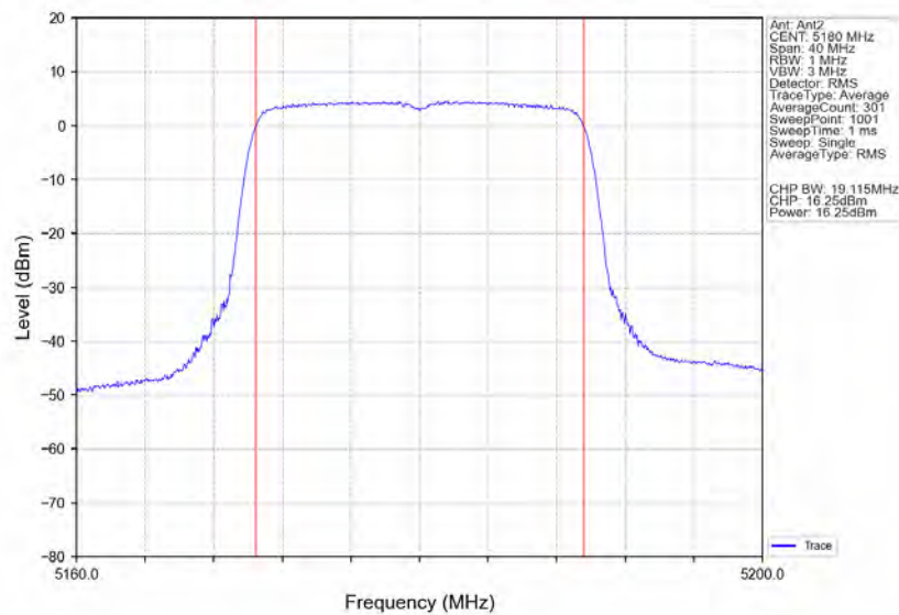
802.11ax(HEW20)_LCH_5180MHz_RU242_Left_Ant2_NTNV
