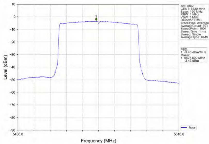
802.11ax(HEW80)_LCH_5530MHz_RU996_Left_MIMO_NTNV
