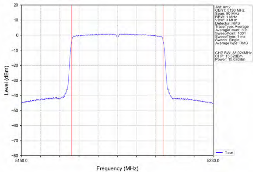
802.11ax(HEW40)_LCH_5190MHz_RU484_Left_Ant2_NTNV
