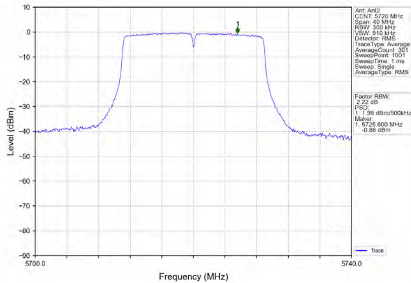
802.11n(HT20)_HCH_5720MHz_MIMO_NTNV
