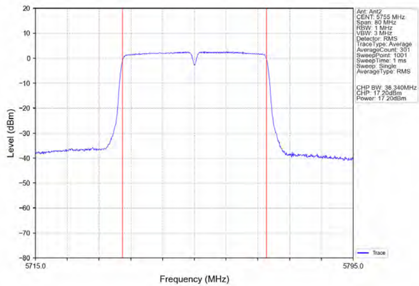
802.11n(HT40)_LCH_5755MHz_Ant2_NTNV
