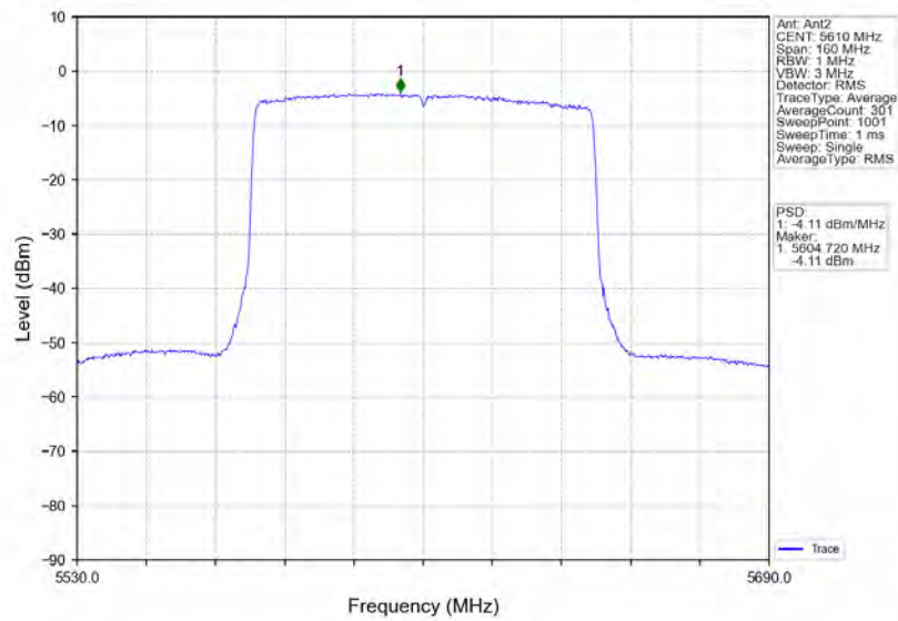
802.11ax(HEW80)_HCH_5610MHz_RU996_Left_Ant2_NTNV
