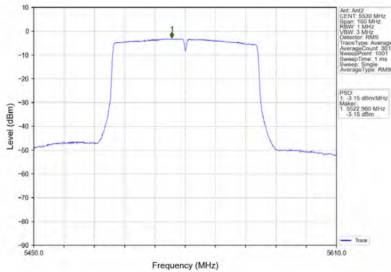
802.11ac(VHT80)_LCH_5530MHz_Ant2_NTNV
