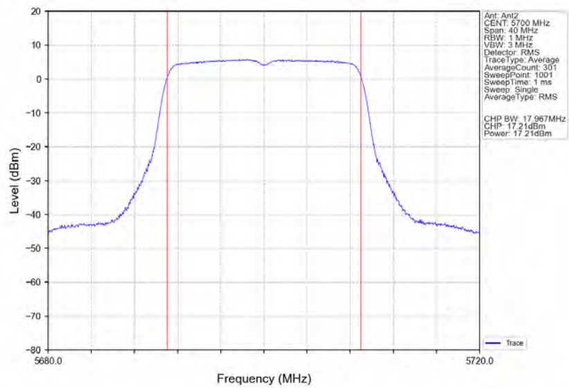
802.11n(HT20)_HCH_5700MHz_Ant2_NTNV
