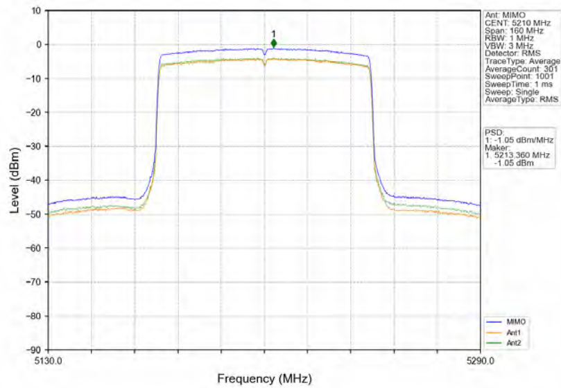
802.11ax(HEW80)_MCH_5210MHz_RU996_Left_MIMO_NTNV
