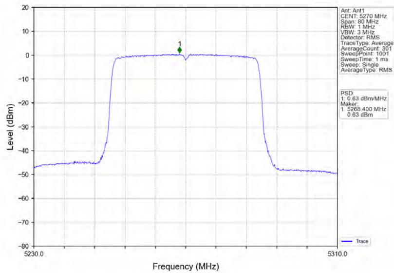
802.11ax(HEW40)_LCH_5270MHz_RU484_Left_Ant1_NTNV
