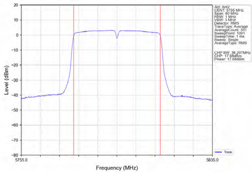
802.11n(HT40)_HCH_5795MHz_Ant2_NTNV
