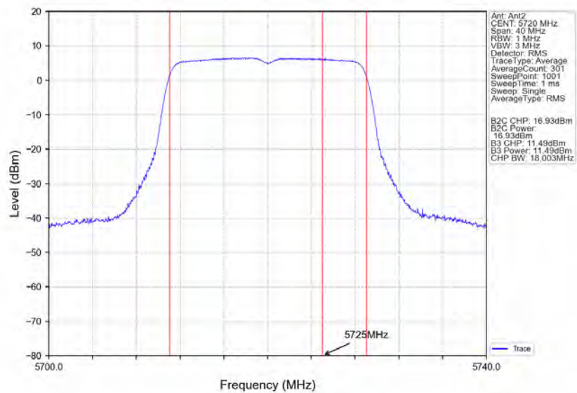
802.11n(HT20)_HCH_5720MHz_Ant2_NTNV
