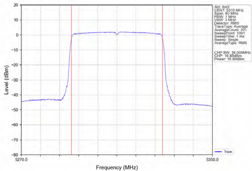
802.11ax(HEW40)_HCH_5310MHz_RU484_Left_Ant2_NTNV
