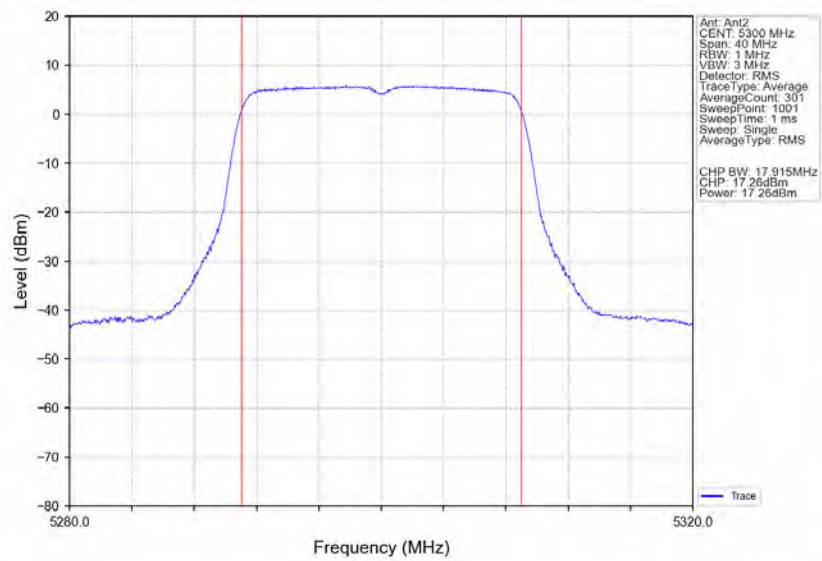
802.11n(HT20)_MCH_5300MHz_Ant2_NTNV
