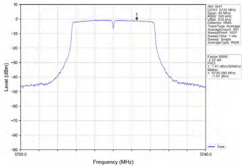
802.11n(HT20)_HCH_5720MHz_Ant1_NTNV
