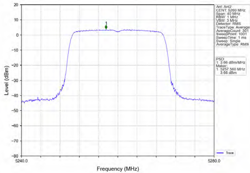
802.11ax(HEW20)_LCH_5260MHz_RU242_Left_Ant2_NTNV
