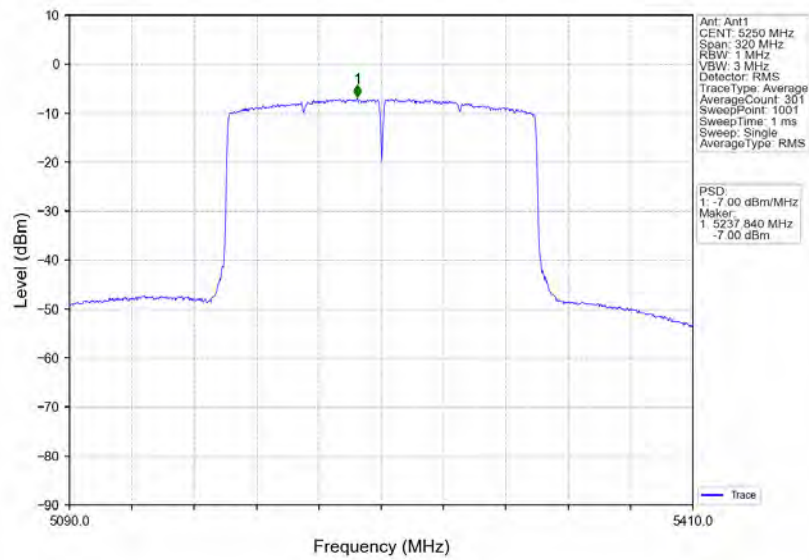
802.11ax(HEW160)_MCH_5250MHz_2xRU996_Left_Ant1_NTNV
