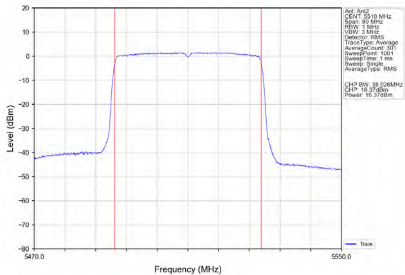
802.11ax(HEW40)_LCH_5510MHz_RU484_Left_Ant2_NTNV
