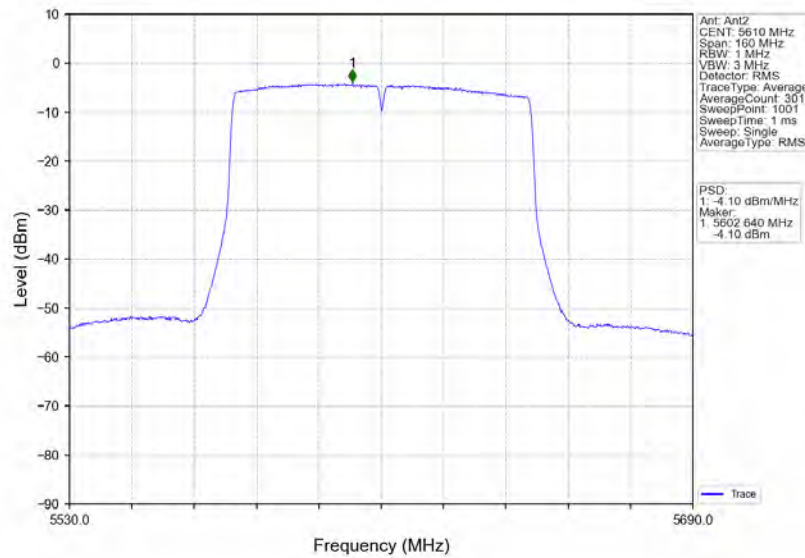
802.11ac(VHT80)_HCH_5610MHz_MIMO_NTNV
