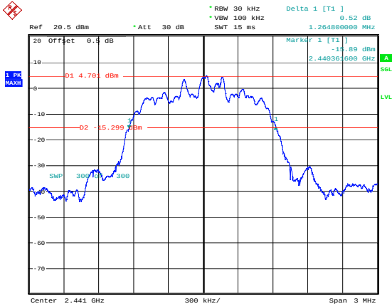
\pi/4 -DQPSK_Middle 1.265MHz
