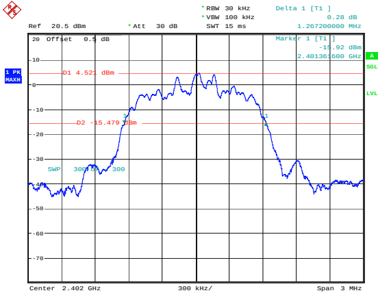
\pi/4 -DQPSK_Low 1.267MHz
