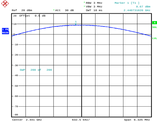
\pi/4 -DQPSK_Middle 8.67dBm
