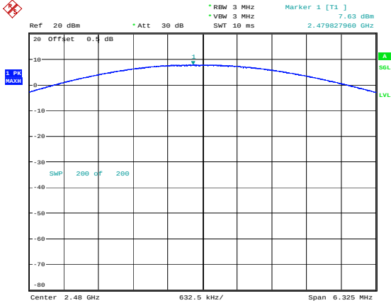
\pi/4 -DQPSK_High 7.63dBm
