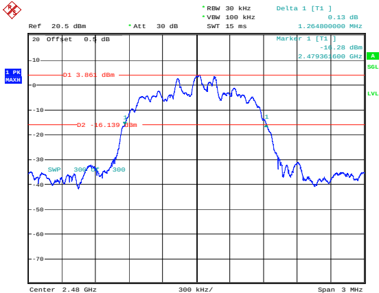
\pi/4 -DQPSK_High 1.265MHz
