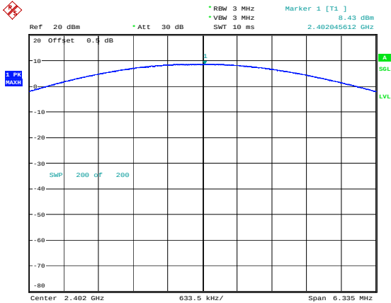
\pi/4 -DQPSK_Low 8.43dBm
