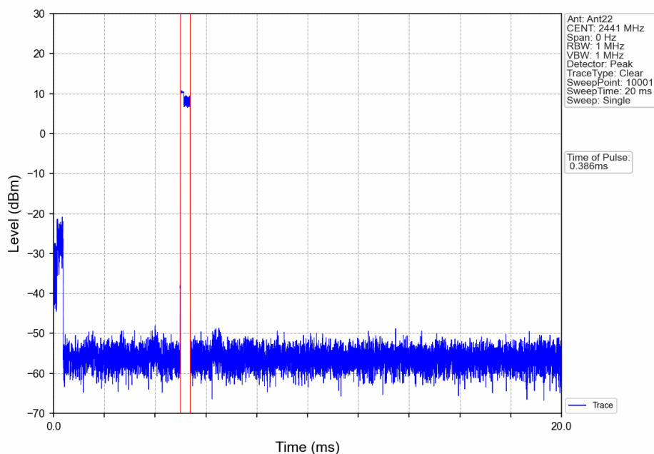
Pi/4DQPSK_2DH1_HOPP_Ant22_NTNV
