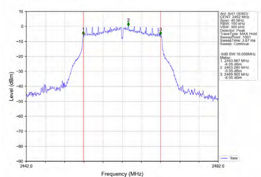
802.11g_HCH_2462MHz_Ant1 (SISO)_NTNV
