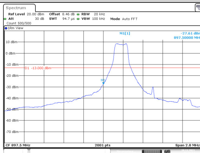
Band8-1.4MHz-QPSK-21632-1-0-Low--27.61-PASS
