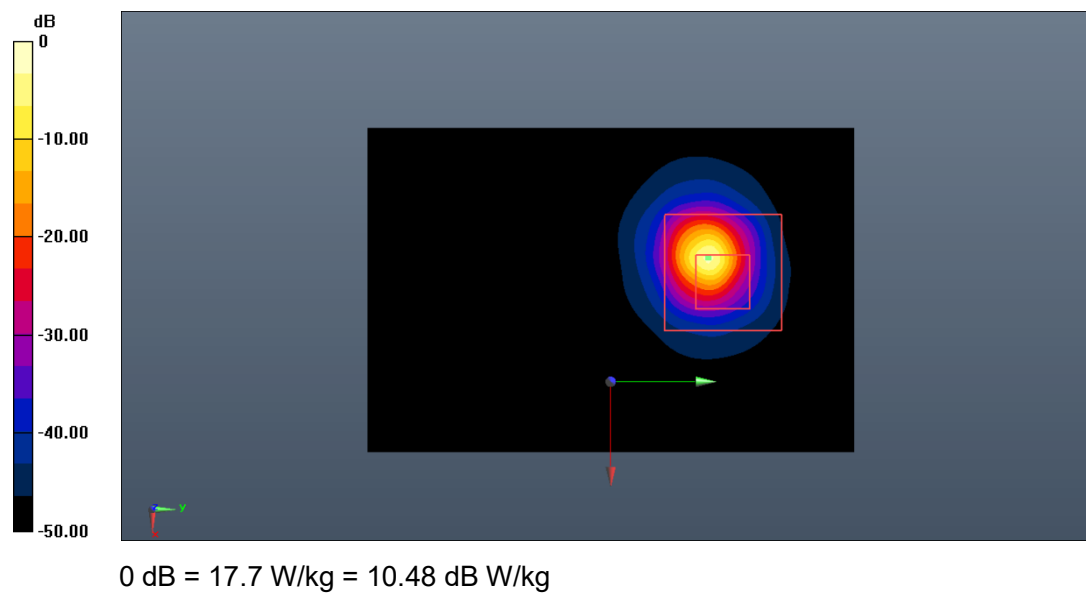
Fig.B.10. Validation 5250MHz 100mW
