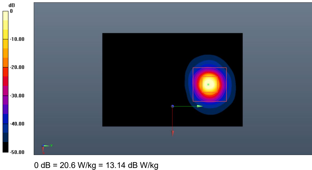
Fig.B.11. Validation 5600MHz 100mW
