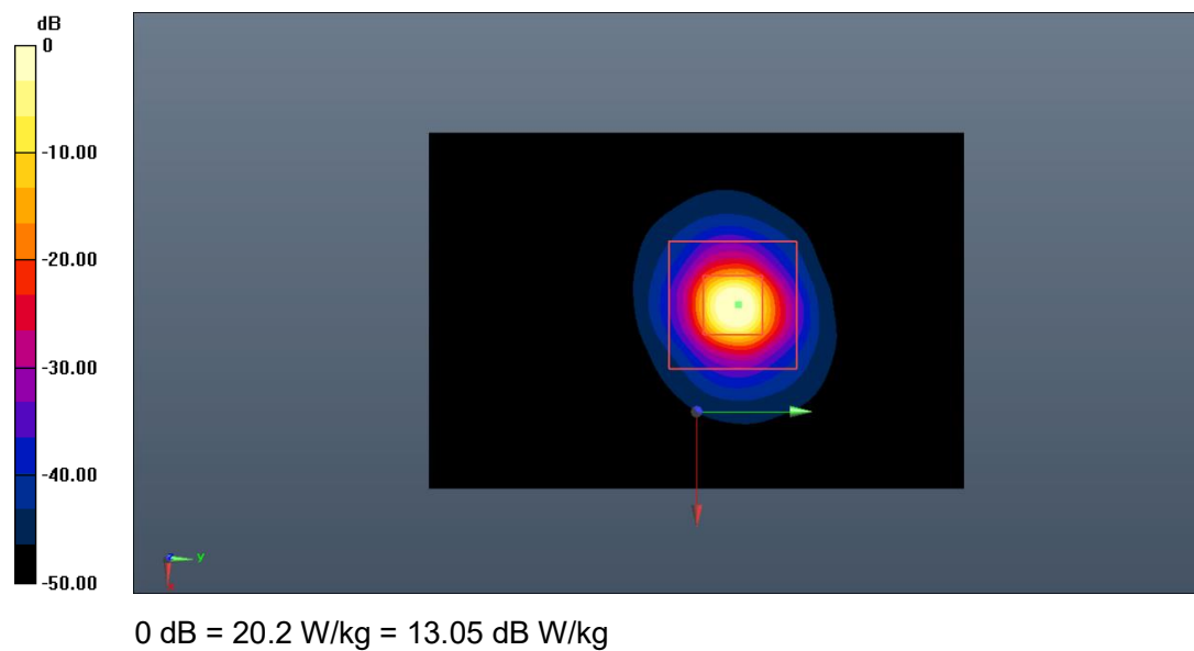
Fig.B.12. Validation 5750MHz 100mW
