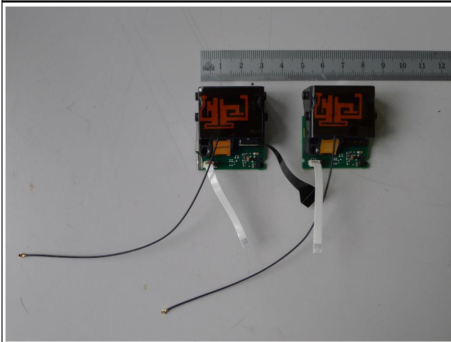
EUT INTERNAL DETAIL (D)
