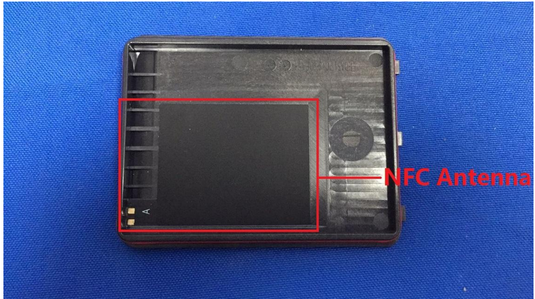
(19) EUT Photo
