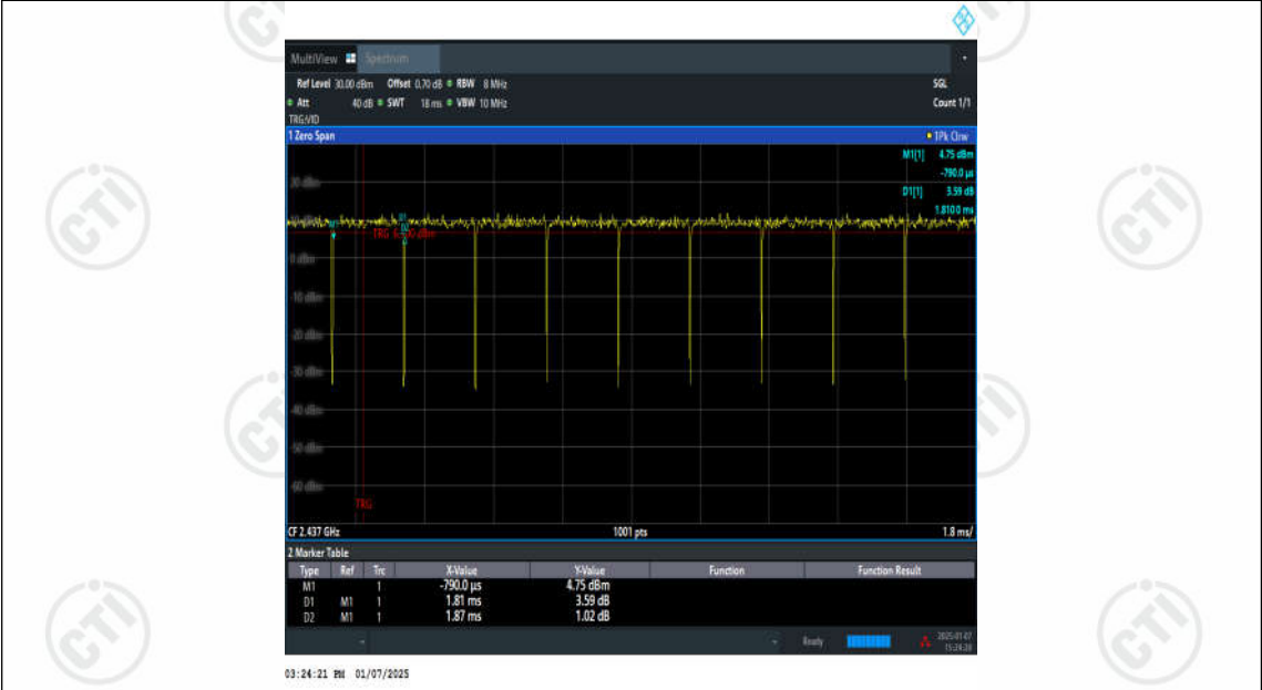
NTNV-11N40MIMO-Ant2-2437
