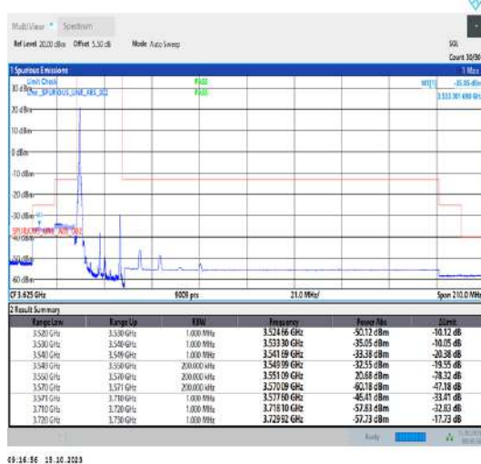
Band42_20MHz_QPSK_43190_1RB#0
