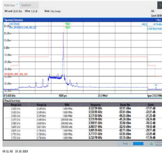
Band42_20MHz_QPSK_43490_1RB#99
