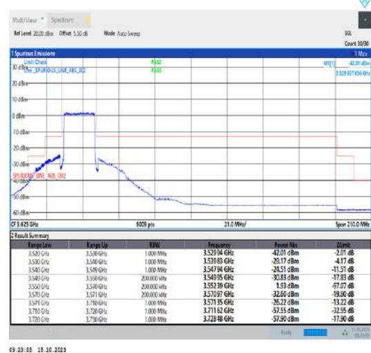
Band42_20MHz_QPSK_43190_100RB#0
