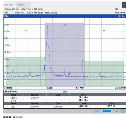
42(3550-3600)-20MHz-QPSK-43190-1RB#0-PASS
