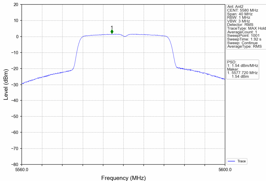
802.11n(HT20)_MCH_5580MHz_MIMO_NTNV
