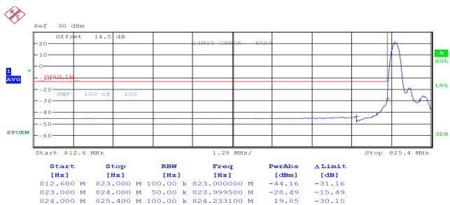
1.4MHz_Low_QPSK_1@0
