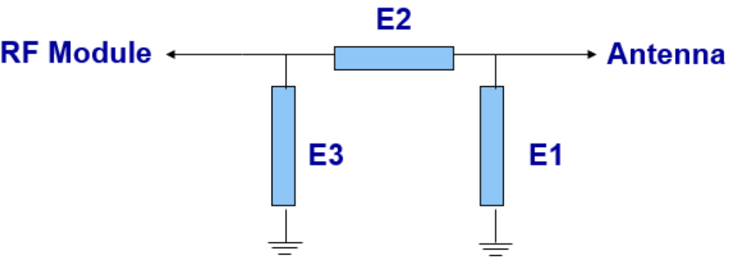
匹配电路
