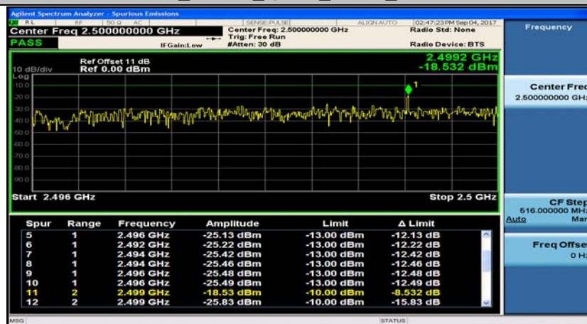
Band7_20MHz_16QAM_20850_100RB#0
