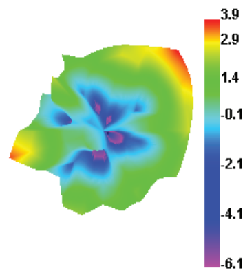
2500.000MHz
