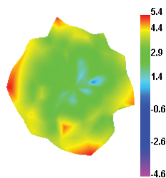
5500.000MHz E1
