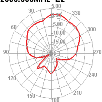
2500.000MHz E2
