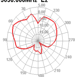
5650.000MHz E2
