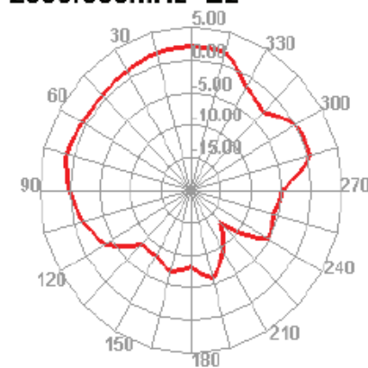
2500.000MHz E2
