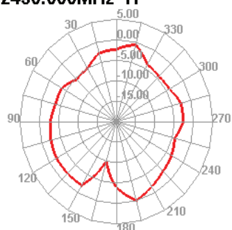
2430.000MHz H
