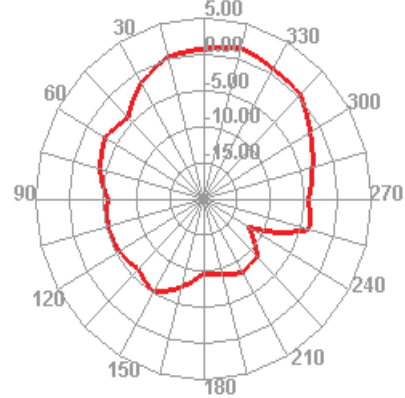
2450.000MHz
