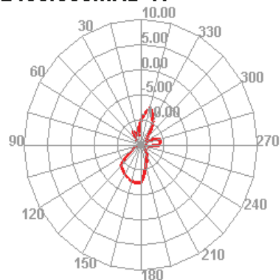
2450.000MHz E2
