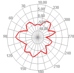
5350.000MHz H
