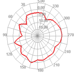
5450.000MHz E2
