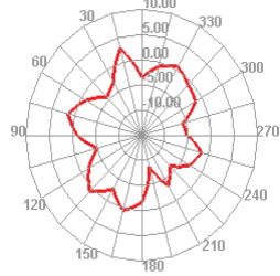
5850.000MHz H
