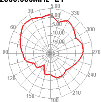
2500.000MHz E1
