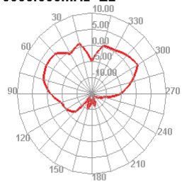
5850.000MHz E2
