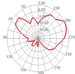
5450.000MHz H
