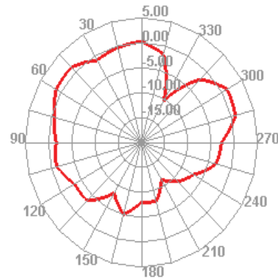
2430.000MHz H
