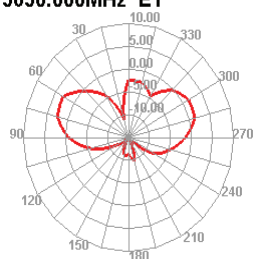
5650.000MHz E1
