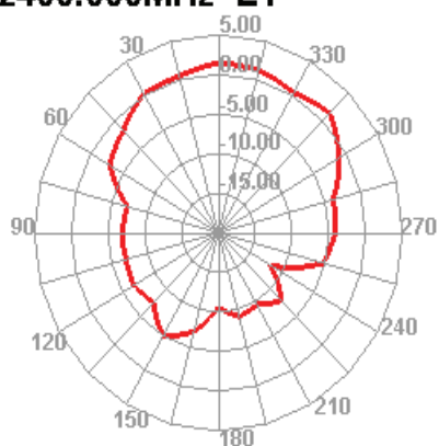
2430.000MHz
