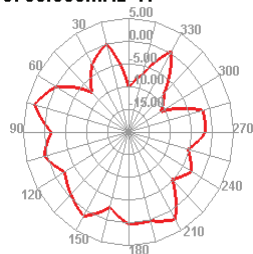
5750.000MHz E2
