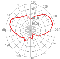
5450.000MHz
