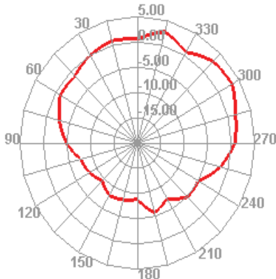
2430.000MHz
