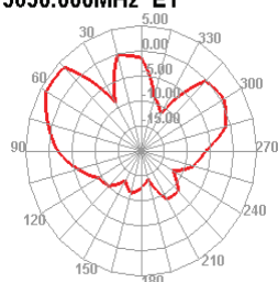
5650.000MHz E1
